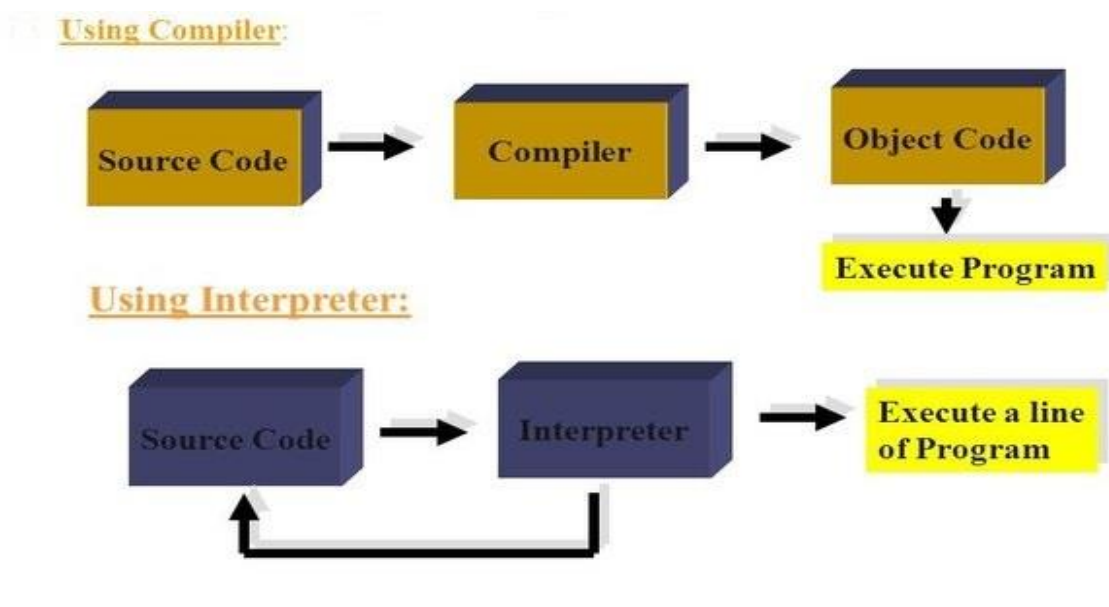
Sl. 2.5. Usporedba ciklusa prevoditelja i interpretera prilikom izvršavanja koda
