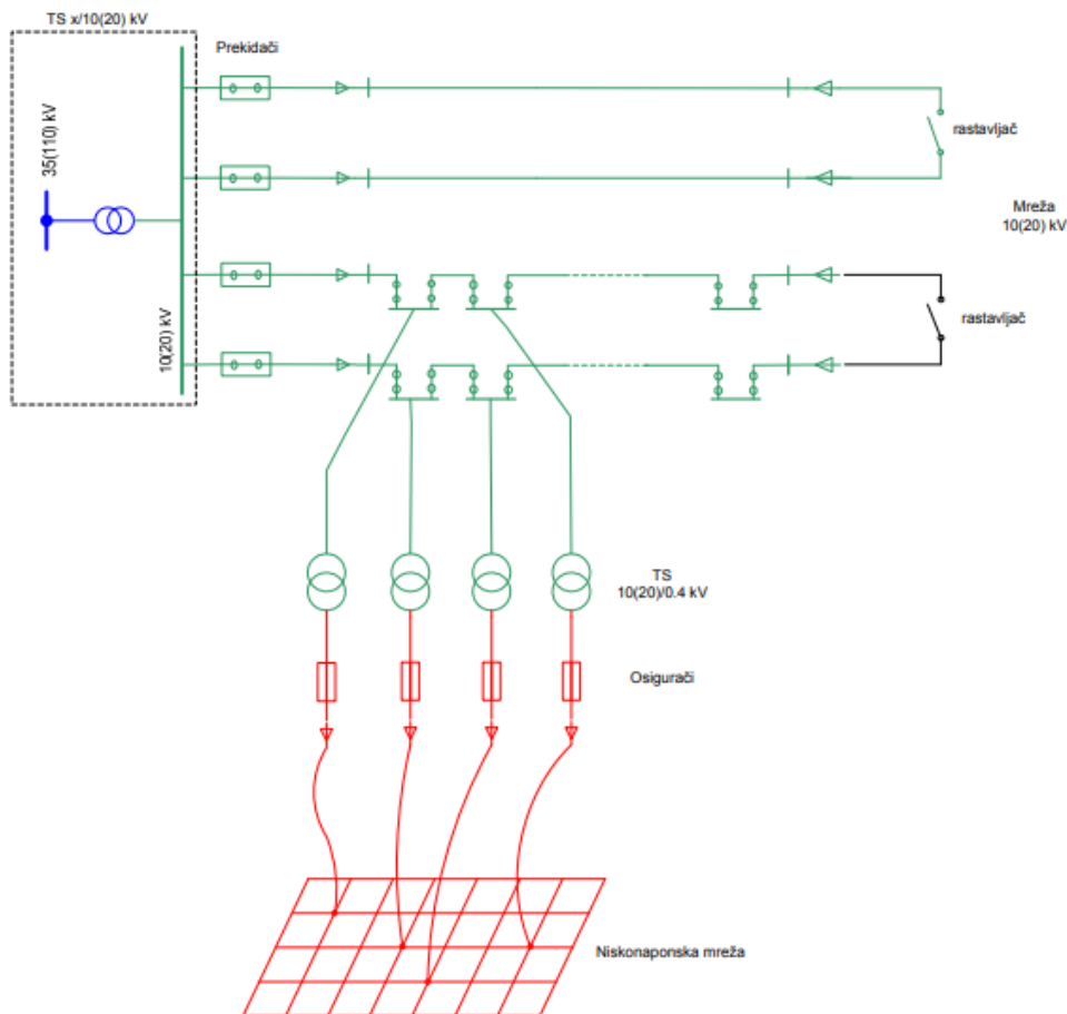
Slika 3.3. Petljasta mreža [13]
