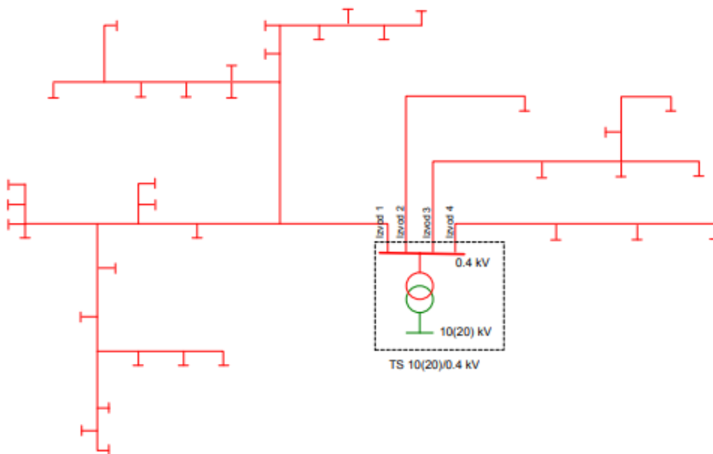
Slika 3.1. Radijalna mreža [13]
