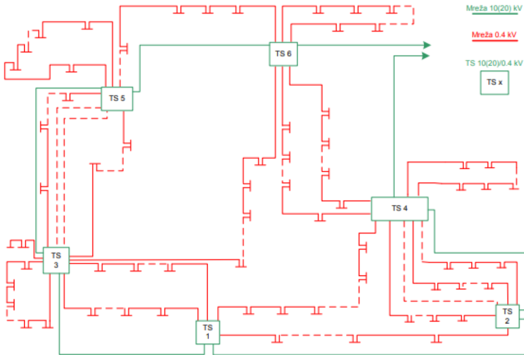
Slika 3.2. Zamkasta mreža [13]
