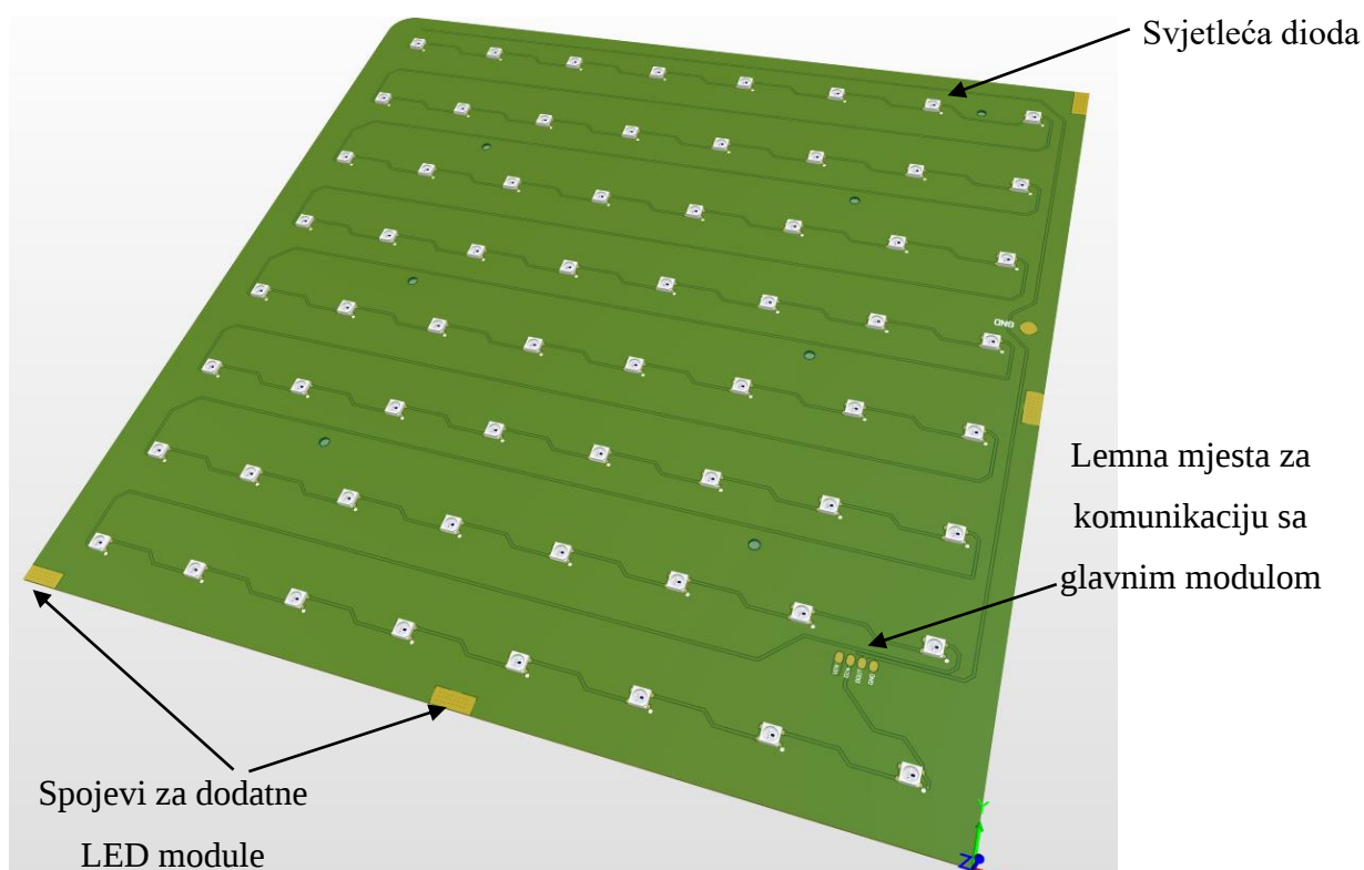
Slika 3.10: LED modul
