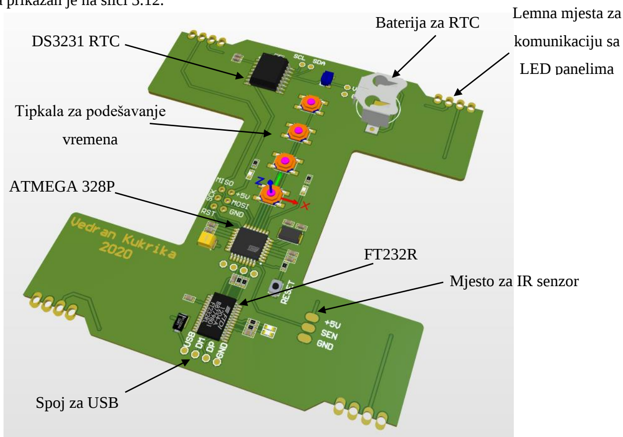
Slika 3.12: Glavni modul
