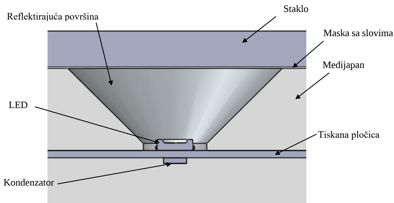
Slika 3.11: Prikaz smještaja svjetleće diode
