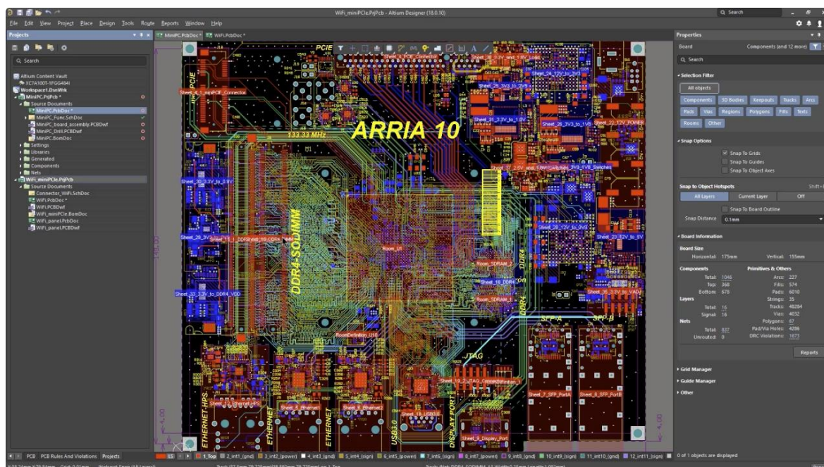
Slika 3.13: Altium Designer
