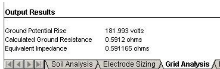
Slika 6.10 Rezultati simulacije „Grid Analysis“
