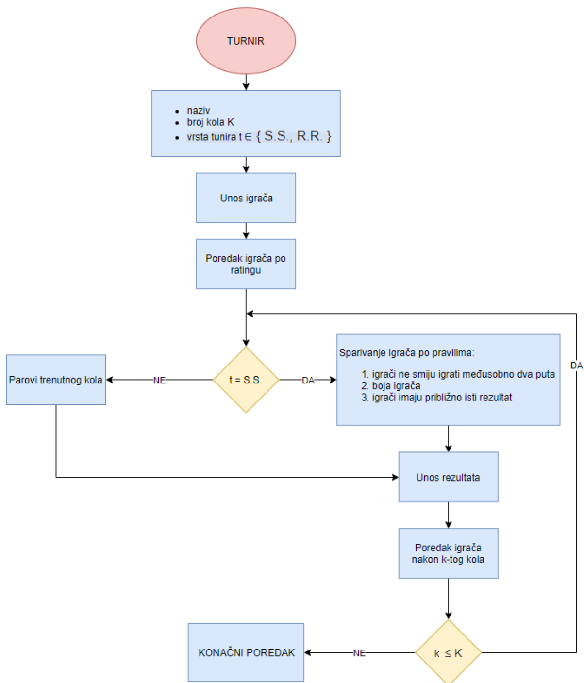
Slika 4.7. – Tok programa
