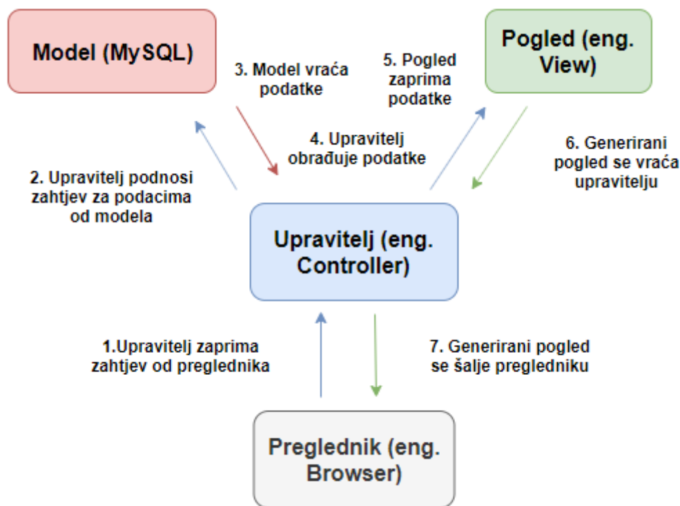
Slika 2.1. – MVC arhitektura u Laravelu
