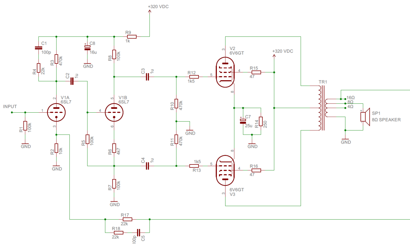
Slika 18 – Shema pojačala
