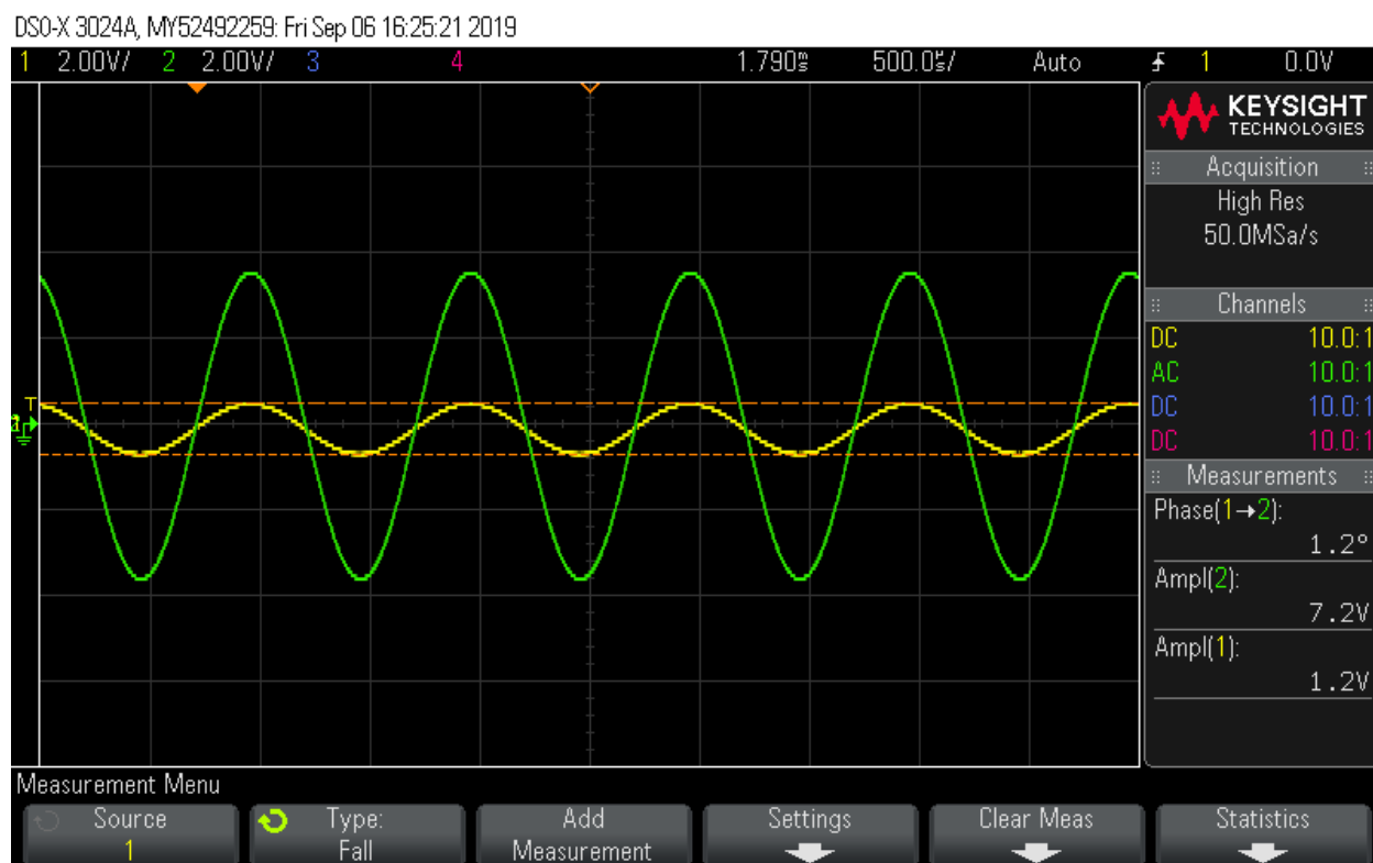
Slika 29 – Slika zaslona osciloskopa pri usporedbi sinala na ulazu pojačala i signala na izlazu pojačala
