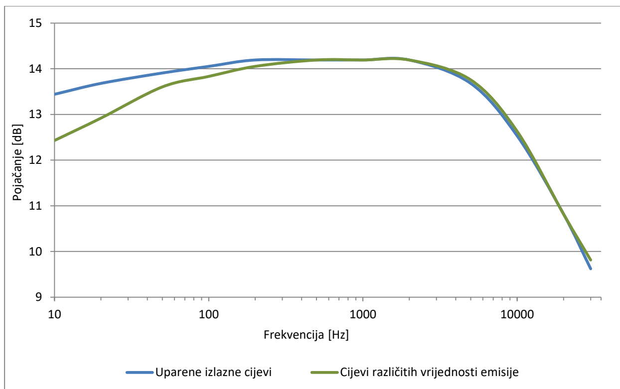
Graf 2 – Mjerene frekvencijske karakteristike bez negativne povratne veze
