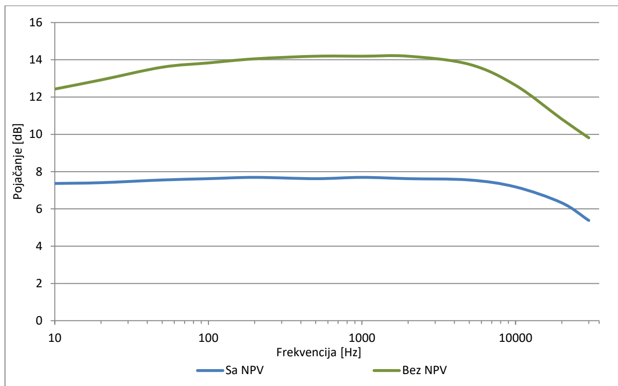
Graf 3 – Usporedba utjecaja NPV na frekvencijsku karakteristiku pojačala
