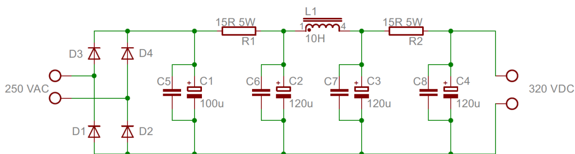
Slika 22 – Shema napajanja
