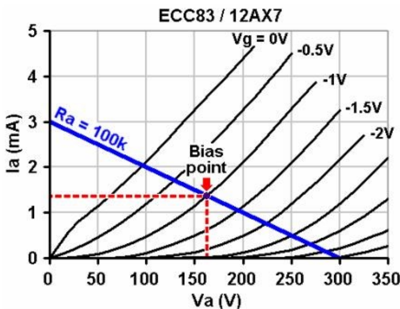
Slika 6 – Radni pravac i statička radna točka [3]
