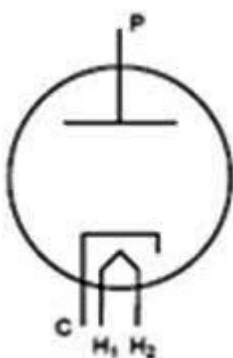
Slika 3 – Simbol diode – anoda (P), katoda (C), grijač ( H_1, H_2 ) [3]
