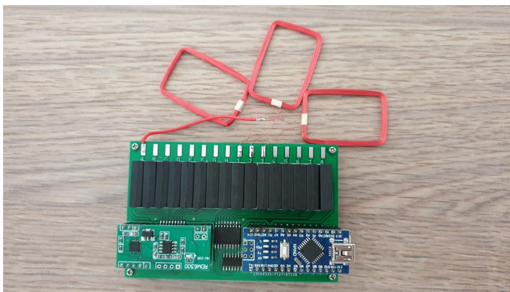
Slika 3.2. Testiranje sklopovlja.
