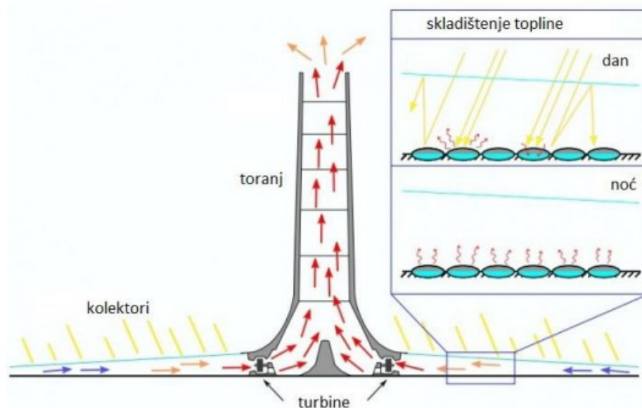
Slika 3.11. Načelo rada solarne dimnjačne elektrane [8]
