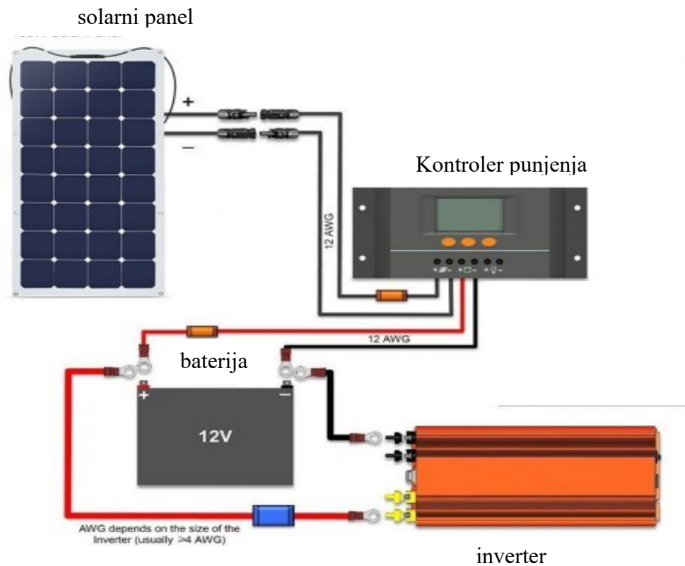
Slika 4.6. Način rada elemenata fotonaponskih sustava [11]
