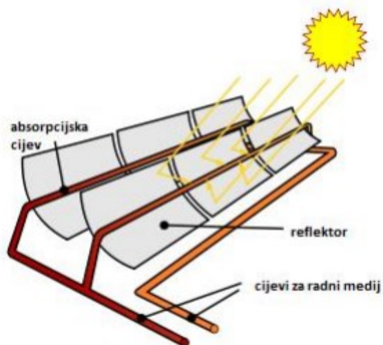
Slika 3.5. Jednostavni prikaz funkcioniranja paraboličnog žljebastog kolektora [5]
