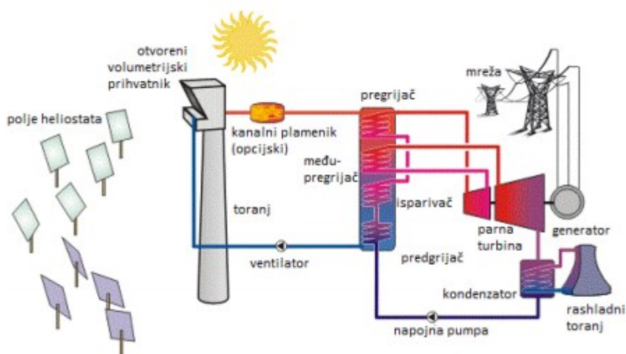
Slika 3.8. Pojednostavljena shema hibridne solarne termoelektrane s otvorenim volumetrijskim prihvatnikom na tornju i poljem heliostata [13]
