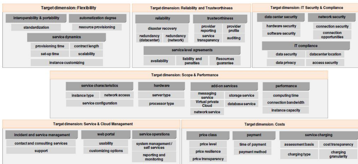
Slika 4.15. Okvir klasifikacije za IaaS [S45]
