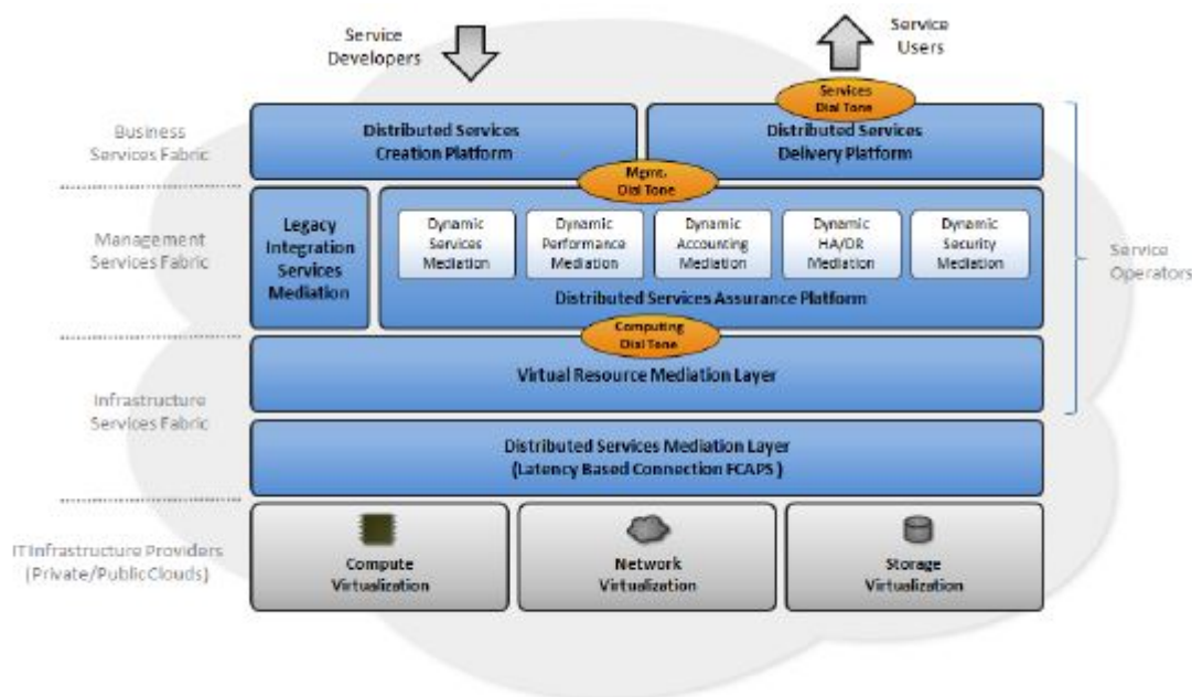
Slika 4.23. Predloženi model referentne arhitekture [S31]
