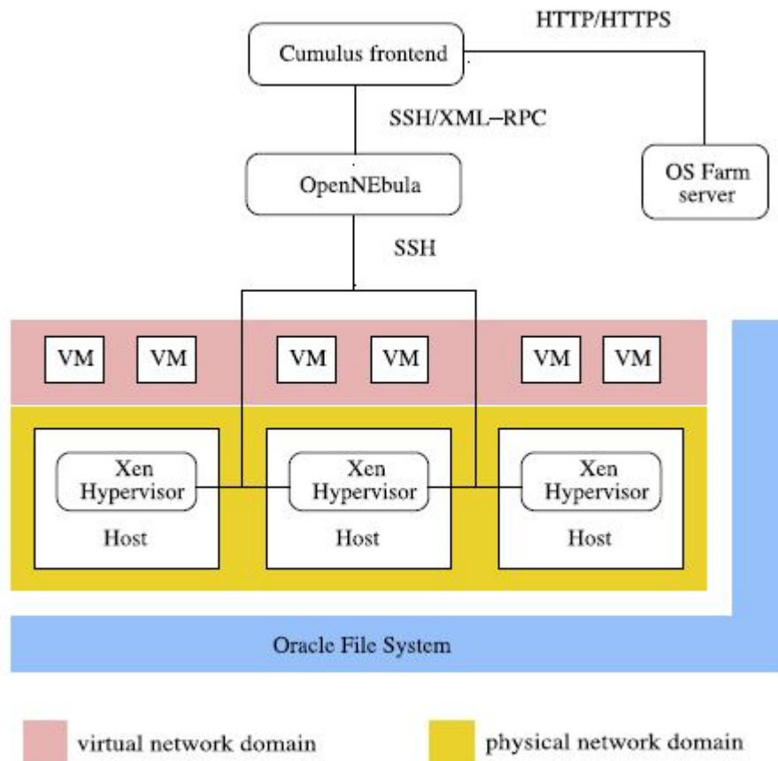
Slika 4.34. Predložena arhitektura Cumulus [S64]
