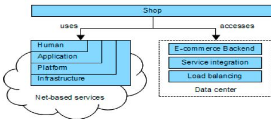
Slika 4.11. Integracija različitih vrsta usluga u web trgovini koristeći oblak aplikaciju [S60]
