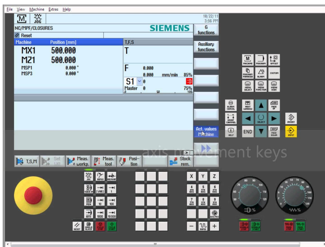
Sl. 3.4. upravljačka jedinica CNC stroja stroja Sinumerik 840D u programskom obliku.
