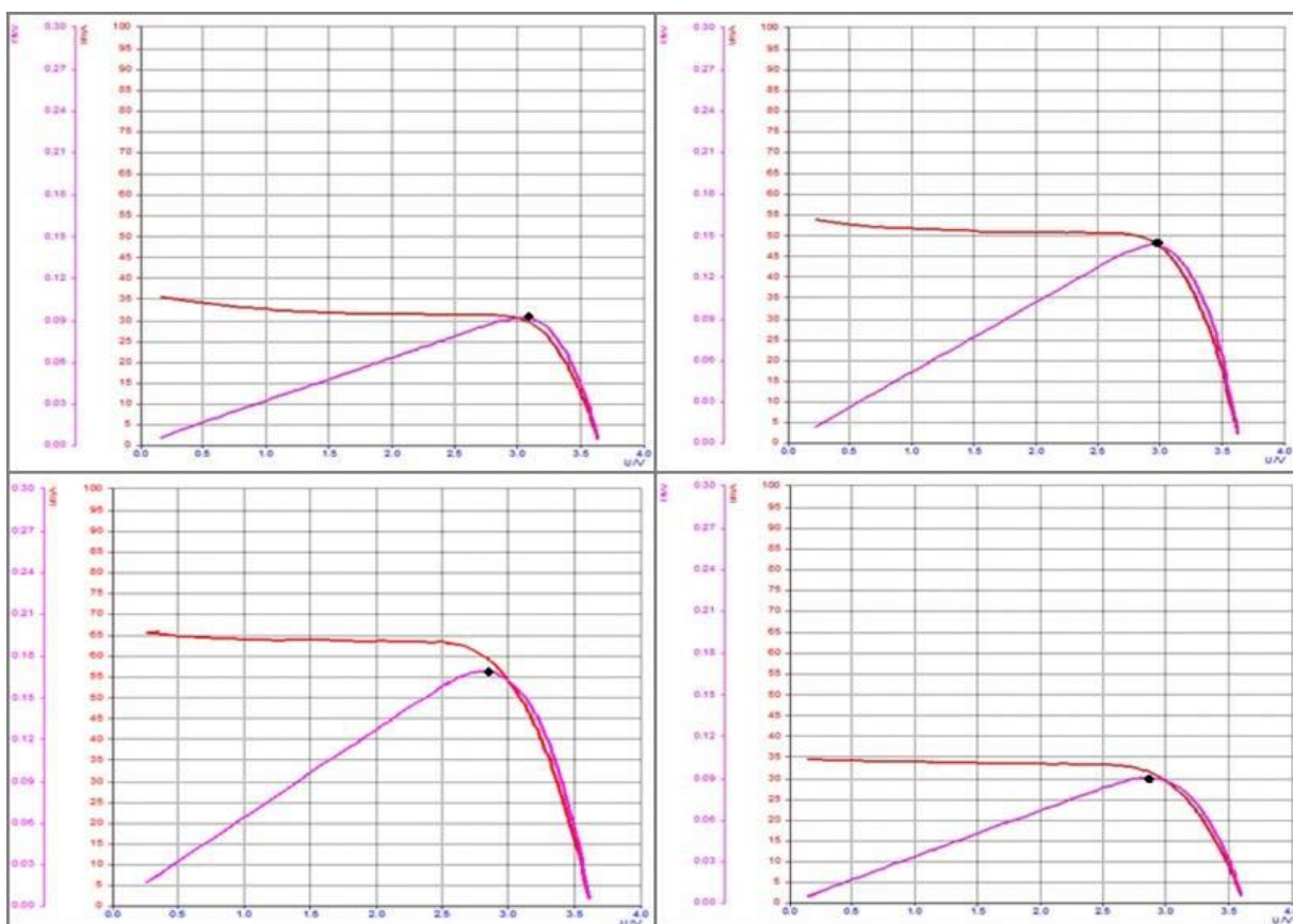
Sl 4.4. Različiti upadni kutevi izvora svjetlosti ( 30^\circ, 60^\circ, 90^\circ, 150^\circ )
