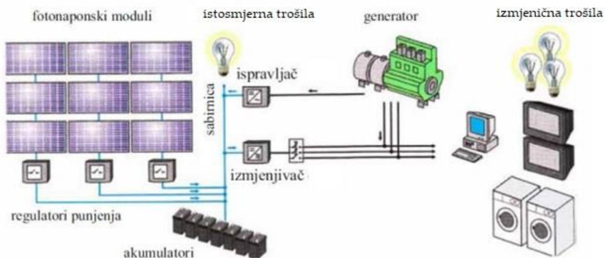
Sl 2.6. Hibridni FN sustav. Izvor: [5]
