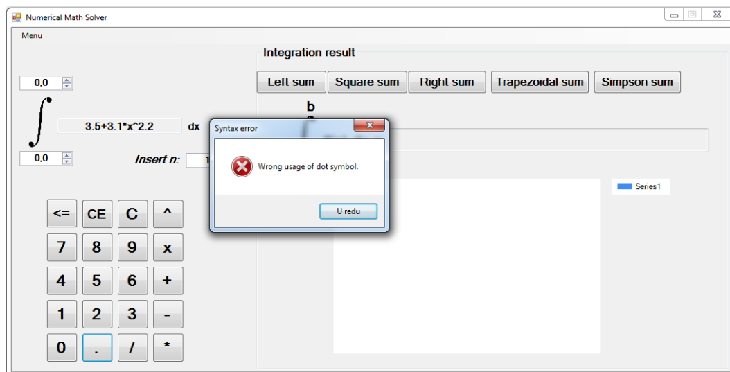
Sl. 4.3 Poruka korisniku pri nekorektnom unosu decimalne točke
