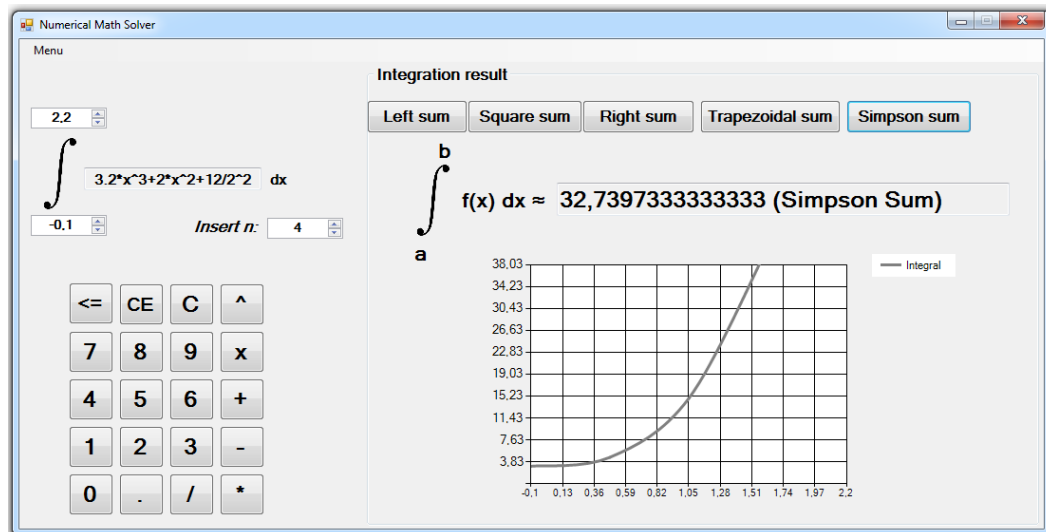
Sl. 4.4 Prikaz rezultata numeričke integracije polinoma Simpsonovom metodom
