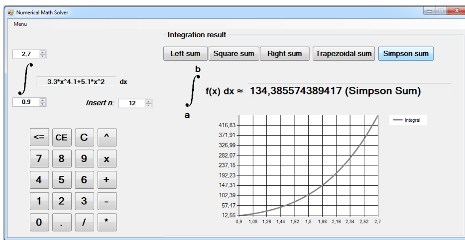
Sl. 5.15 Rezultat integracije Simpsonovom formulom (Rezultat: 134.385)
