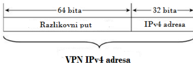
Slika 5.3. VPNv4 adresa [45]
