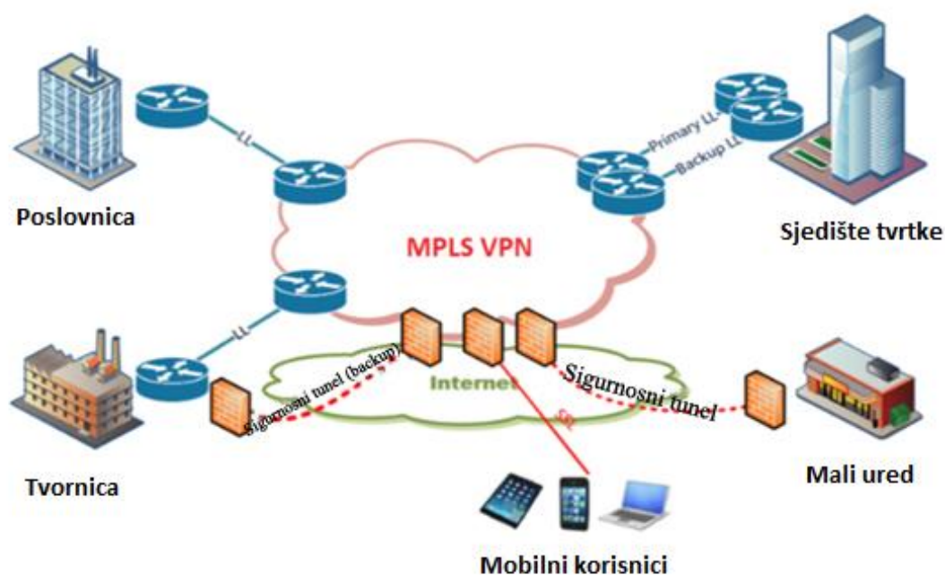
Slika 5.1. MPLS VPN [40]
