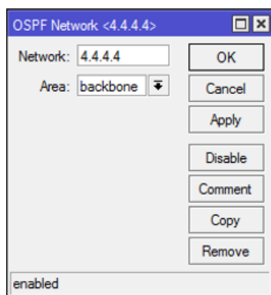
Slika 8.51. Mreža 4.4.4.4
