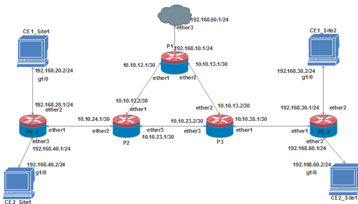
Slika 8.1: Mrežna topologija
