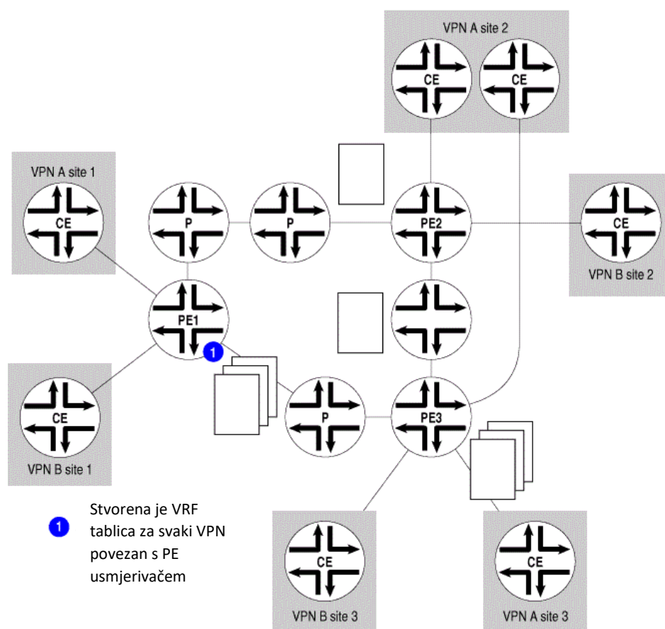
Slika 5.5 VRF tablice [47]
