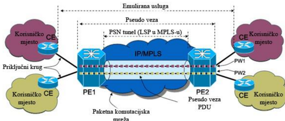
Slika 5.8. PWE3 model [50]
