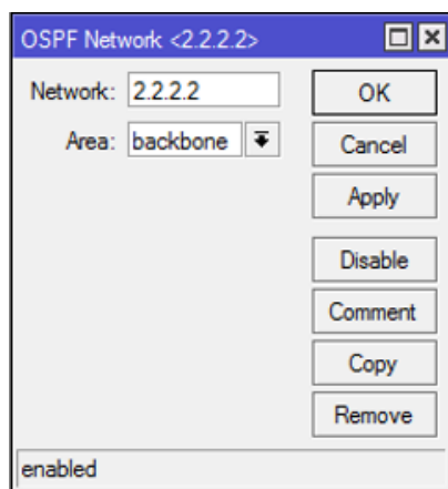
Slika 8.35. Mreža 2.2.2.2
