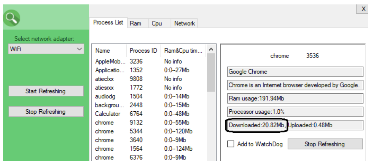
Sl. 5.10 Prikaz količine preuzetih podataka od strane izabranog procesa
