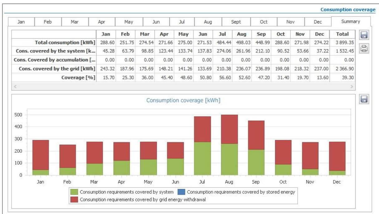
Slika 4.9. Pokrivanje potreba kućanstva
