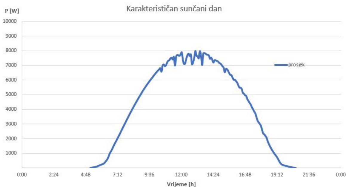
Slika 3.8. Sunčani karakterističan dan elektrane ETFOS 1 [14].
