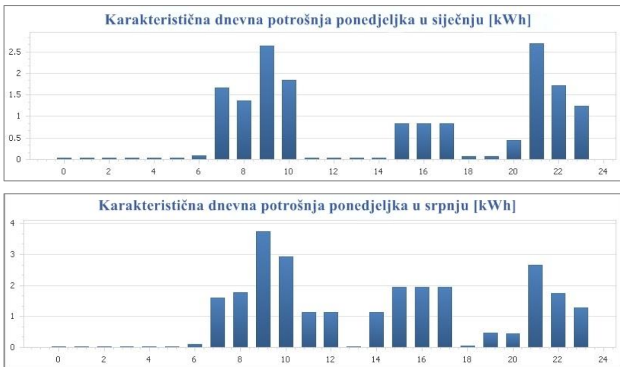
Slika 4.2. Usporedni prikaz karakterističnog ponedjeljka u kućanstvu zimi i ljeti
