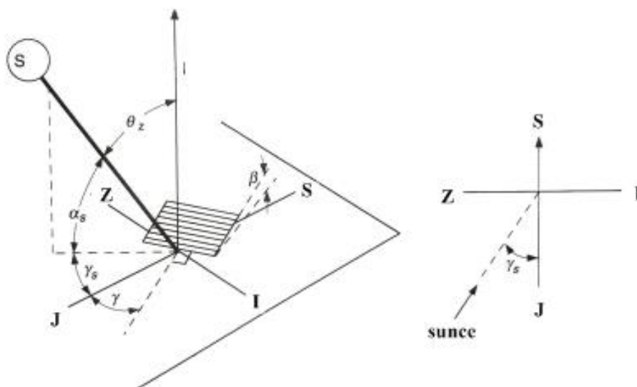
Slika 3.4. Kutovi upada zraka i položaja modula [11]
