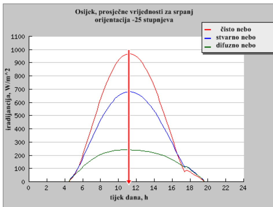
Slika 3.12. Ozračenost FN modula sa orijentacijom 25^\circ istočnije
