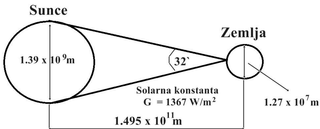
Slika 2.2. Osnovne relacije Sunca i Zemlje te prostorni kut upada Sunčeve energije na Zemlju.
