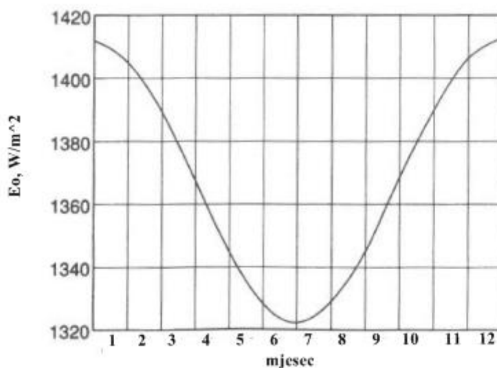
Slika 3.3. Sunčevo zračenje kroz godinu [7]
