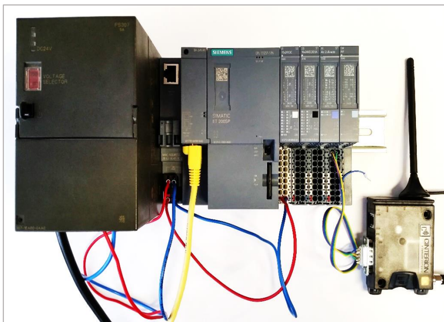
Slika 2.3. Korištena oprema.
