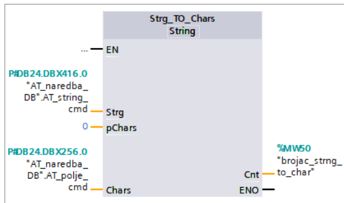
Slika 4.6. Funkcijski blok za pretvaranje niza znakova u polje znakova u TIA portalu v14.
