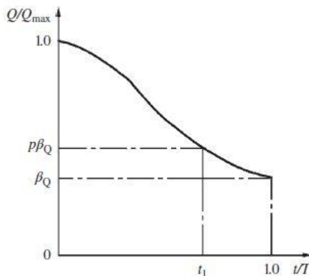
Sl. 3.4. p > 1 , Bepovratni prijenos jalove snage
