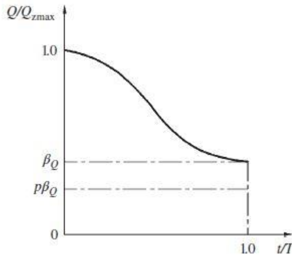
Sl. 3.3. Podkomenzacija, p < 1
