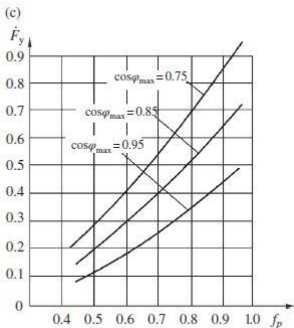
Sl. 3.6. Izračun krivulje godišnjih gubitaka električne energije u iznosu od 35 do 110 kV dalekovoda : (a) \beta_y = 0.20 ; (b) \beta_y = 0.30 ; (c) \beta_y = 0.40 ; (d) \beta_y = 0.50
