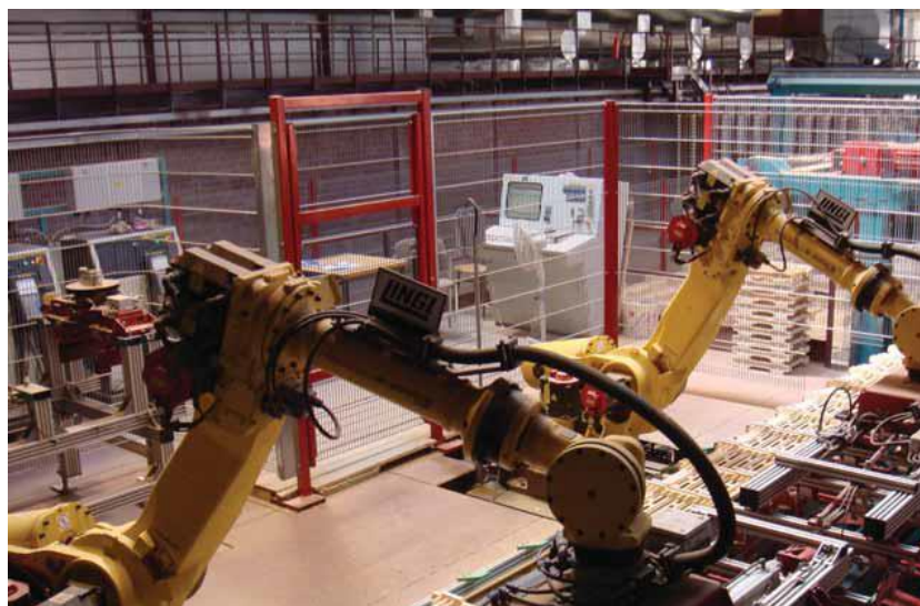
Slika 4.35. Slaganje crijepa na paletu
