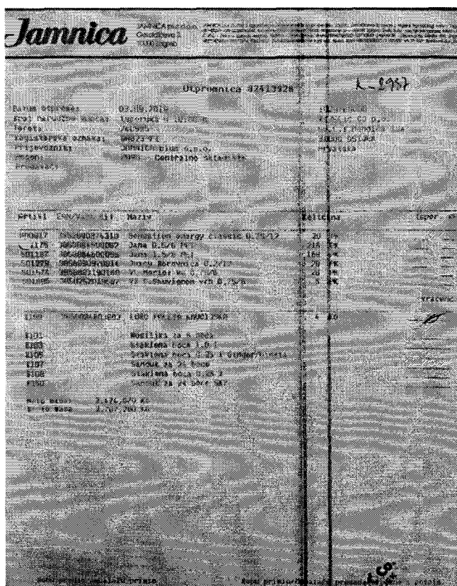
Slika 7: primjer otpremnice
