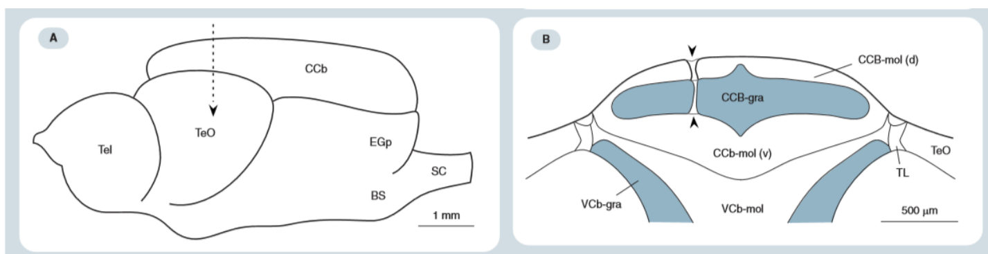
Slika 2. A) postrani pogled na mozak A. leptorhynchus . CCB – corpus cerebelli se nalazi na vrhu mozga i prekriva sve osim telencefalona (Tel), pa se lezije lako vrše na tom dijelu mozga bez oštećenja drugih dijelova. B) poprečan prerez kroz corpus cerebelli napravljen na mjestu koje prikazuje strelica na slici A), strelice na slici B) prikazuju mjesto lezije, proteže se preko molekularnog sloja dorzalnog dijela (CCB-mol(d)) i granularnog sloja (CCB-gra) (Zupanc, Zupanc, 2006b)
