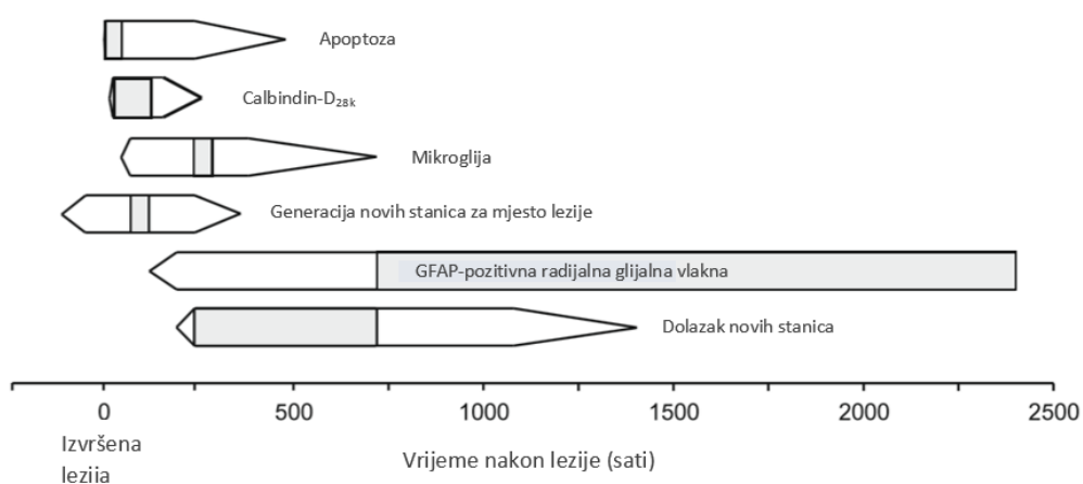
Slika 15 Shematski prikaz događaja uključenih u regeneraciju neuralnih stanica na mjestu ozljede mozga. 1. apoptoza stanica na i u blizini mjesta lezije. 2. ekspresija calbindin- D_{28k} . 3. povećanje gustoće mikroglija. 4. generacija novih stanica koje odlaze na mjesto ozljede, stanice generirane prije ozljede su također uključene u proces. 5. povećanje gustoće GFAP-pozitivnih radijalnih glijalnih vlakana na i u blizini mjesta lezije. 6. dolazak novih stanica na mjesto lezije. Osjenčana područja prikazuju vrhunac svakog događaja. Prije osjenčanih područja su razdoblja povećanja efekta događaja, a nakon su područja smanjenja. (preuzeto i prilagođeno iz Zupanc, 2008)
