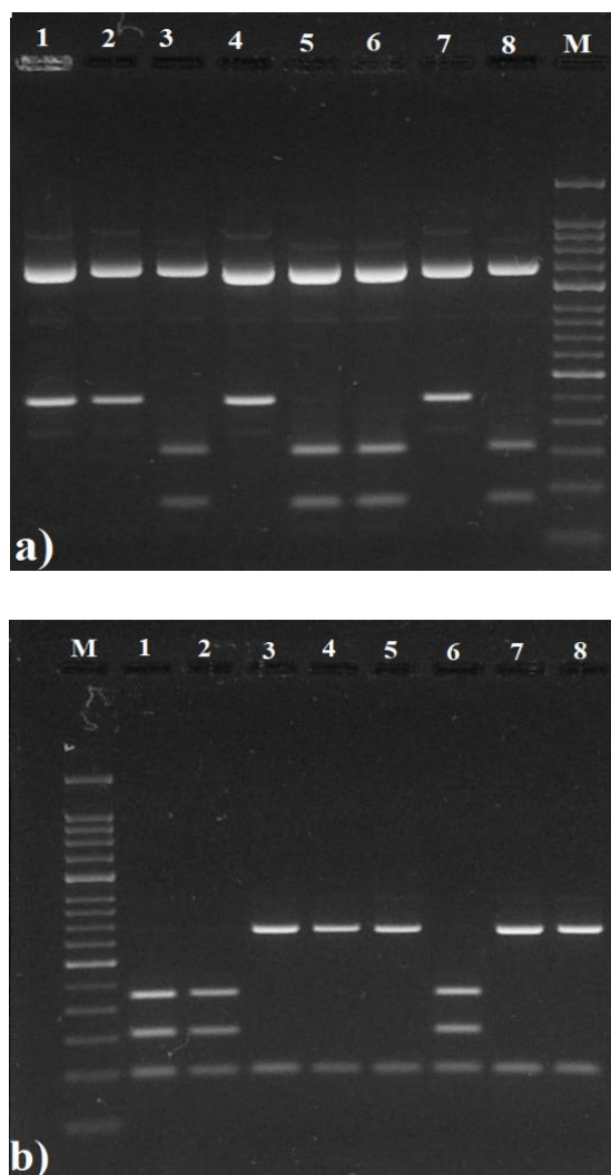
Slika 2. Restrikcijski elektroforetski obrazaci izolata O. novo-ulmi s lokaliteta Nova Kapela dobiveni cijepanjem umnoženog odsječka gena cu pomoću enzima Hph I (a) i cijepanjem umnoženog odsječka gena col1 pomoću enzima Bfa I ( Fsp BI) (b): 1 – NK8, 2 – NK11, 3 – NK14, 4 – NK18, 5 – NK21, 6 – NK22, 7 – NK23, 8 – NK24, M-50 bp (DNA Ladder).
