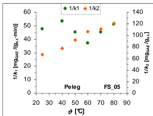
Slika 4.9. Utjecaj temperature ( \vartheta ) ekstrakcije na recipročne vrijednosti parametara ( 1/k_1 , 1/k_2 ) neeksponencijalnog Pelegova modela
