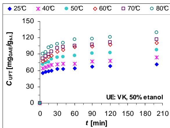
Slika 4.5. Ovisnost masenog udjela ukupnih fenolnih tvari ( C_{UFT} ) u ekstraktima sjemenki grožđa FS_05 o vremenu ( t ) kruto-tekuće ekstrakcije za različite temperature ekstrakcije (eksploimentalni podaci)
