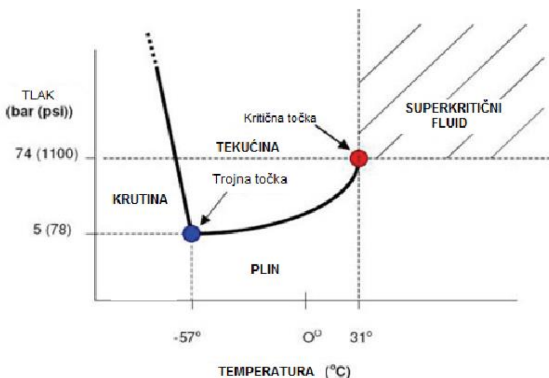
Slika 5 Fazni dijagram za CO 2 (Panak Balentić i sur., 2017)
