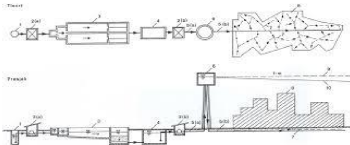
Slika 1. Definicijaska shema vodoopskrbnog sustava (Vuković, 2016)
