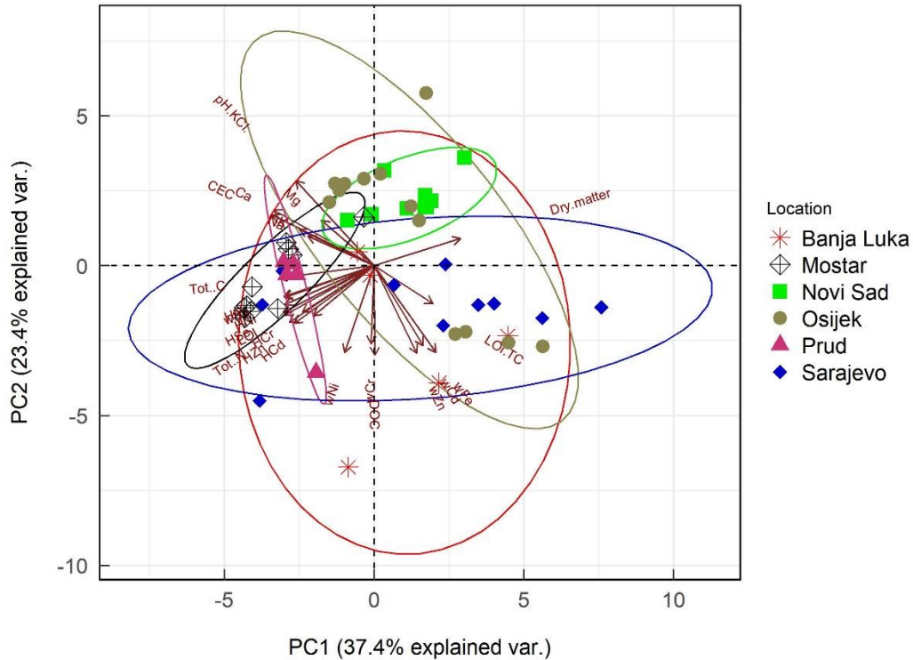
Slika 2. Biplot glavnih komponenti 1 i 2 iz PC analize varijacija među šest lokacija s različitim svojstvima tla. Strelice predstavljaju svojstvene vrijednosti (eng. “eigenvalues”) svakog od 24 odabrana parametra tla. Izvor: Galić i sur., 2023.
