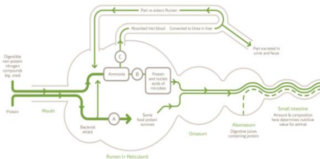
Slika 4. Ciklus dušika
