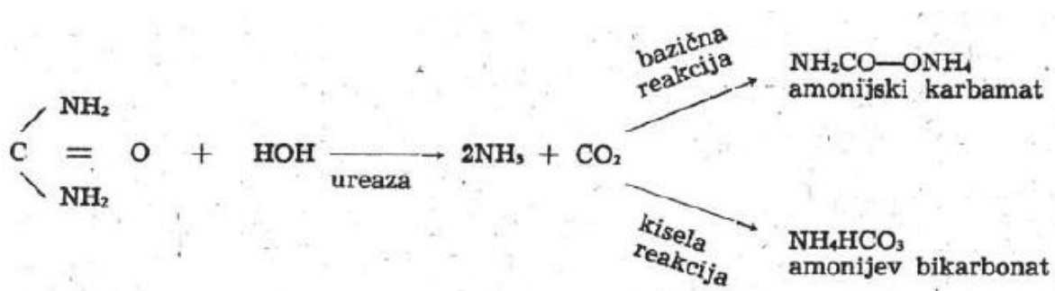
Slika 6. Razgradnja uree
