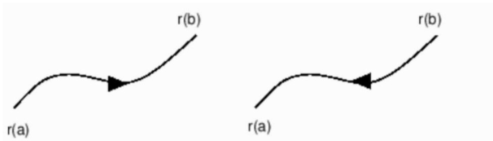
Slika 2: Krivulja \Gamma
