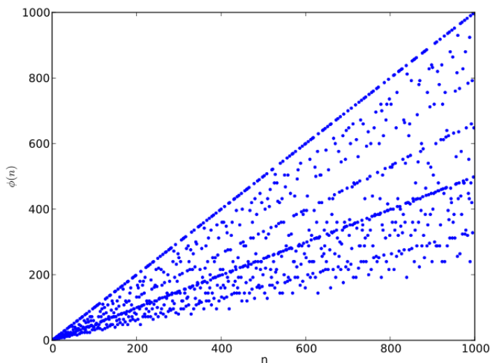
Slika 2: Graf koji prikazuje prvih 1000 vrijednosti Eulerove funkcije
