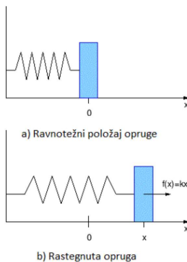
Slika 7: Hookeov zakon
