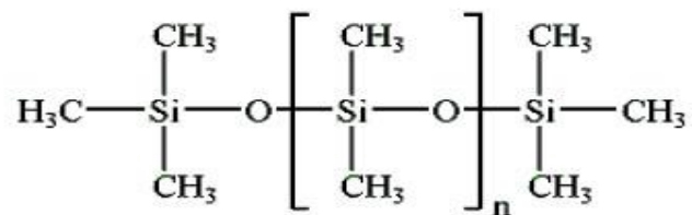
Slika 2. Struktura polidimetilsiloksana
