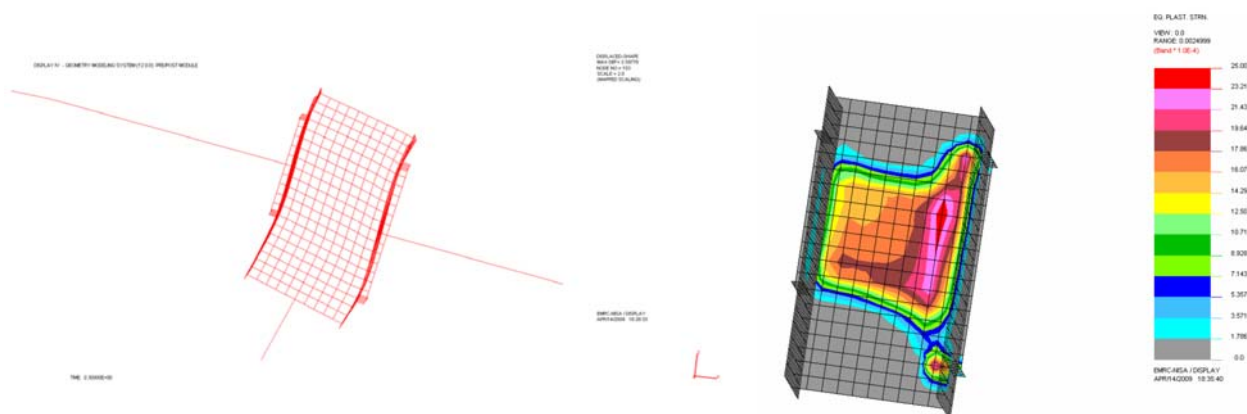
Slika 14. Nelinearne deformacije i plastifikacija hrptenog panela
