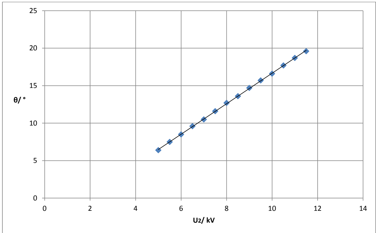
Graf 5: Ovisnost kuta torzije o naponu na drugoj kuglici ( \theta - U_2 )
