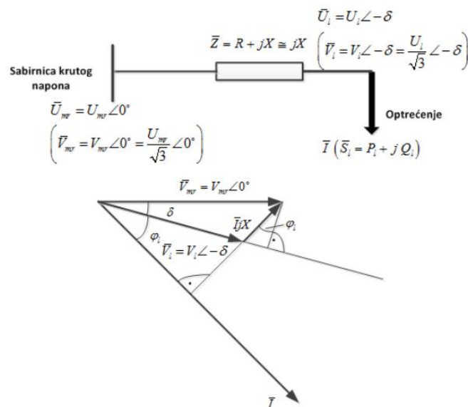
Slika 3.2: Jednostavni prijenosni sustav i pripadajući fazorski dijagram
