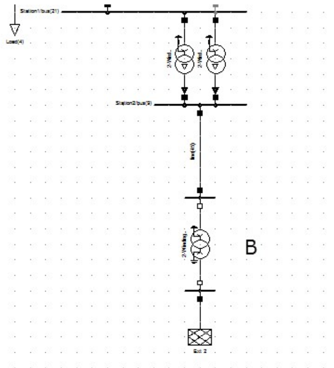
Sl.4.31. Prikaz isključenog transformatora nakon t = 150 ms
