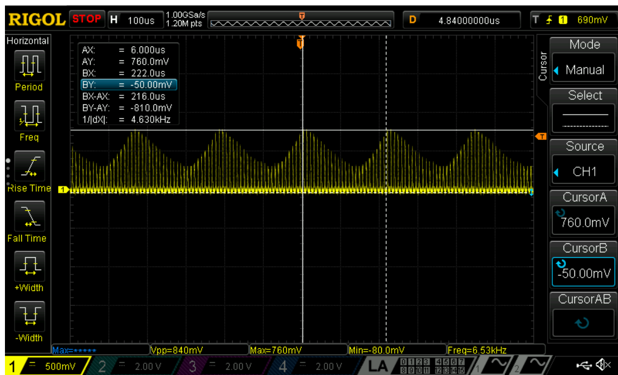
Sl. 4-13 Oscilogram izlaza naponskog sljedila
