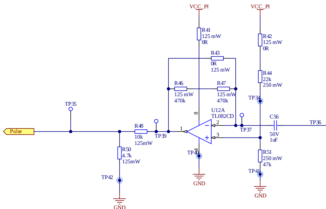
Sl. 5-11 Shema derivatora PI detektora
