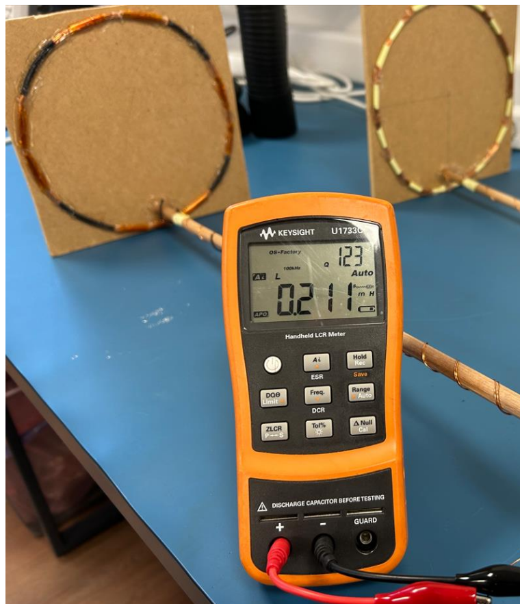
Sl. 4-3 Mjerenje induktiviteta BFO zavojnice RLC-metrom
