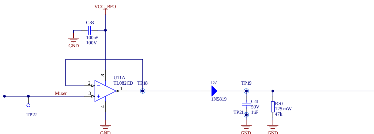
Sl. 4-12 Shema amplitudnog demodulatora
