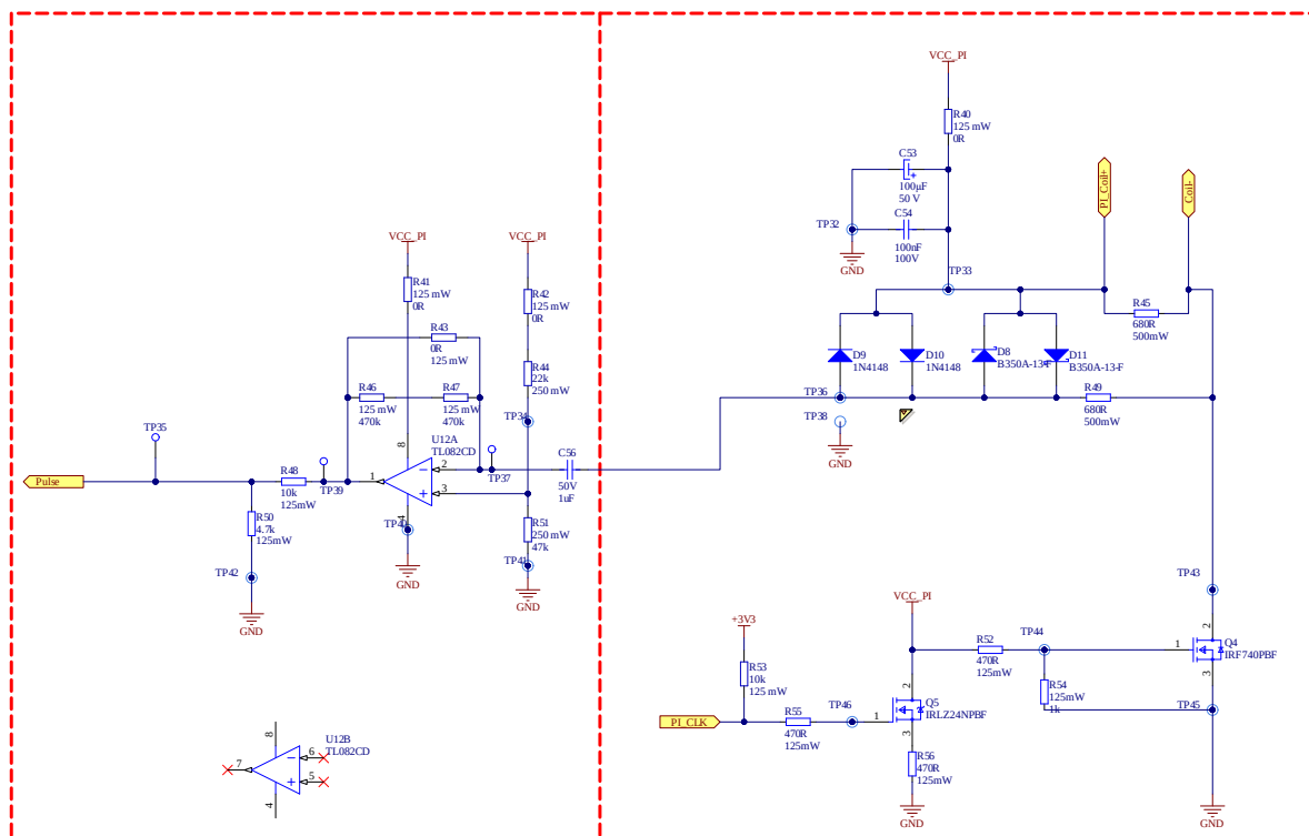
Sl. 5-2 Shema PI detektora
