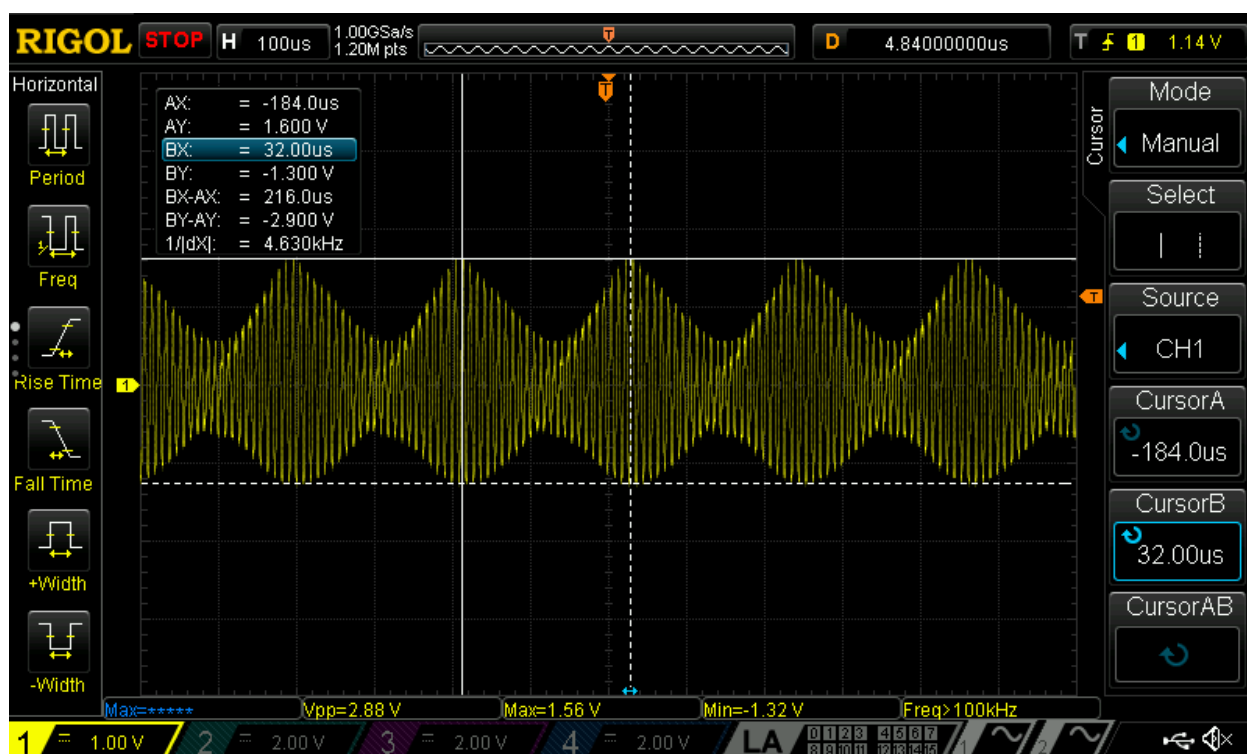
Sl. 4-11 Oscilogram izlaznog signala frekventijskog miksera
