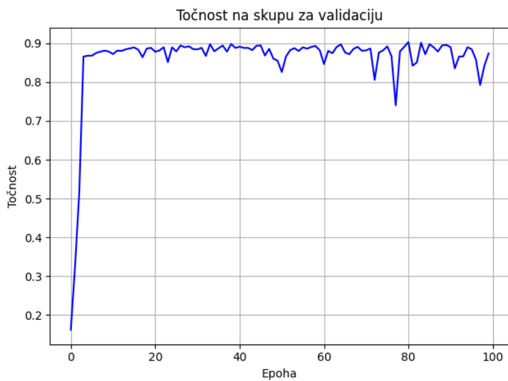
Slika 5.22: Graf točnosti na validacijskom skupu kroz epohe.
