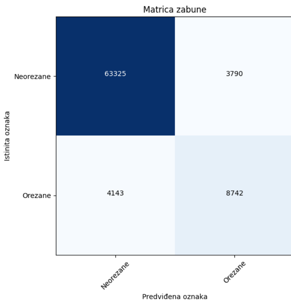
Slika 5.25: Matrica zabune.
