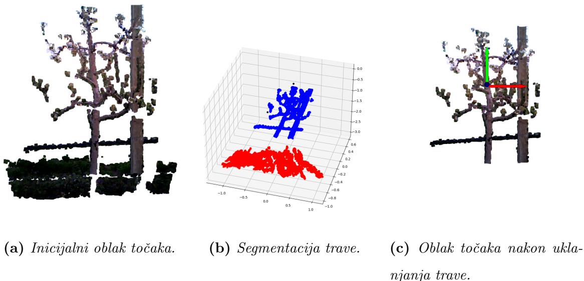
Slika 4.11: Proces uklanjanja trave iz oblaka točaka pomoću K-means algoritma.
