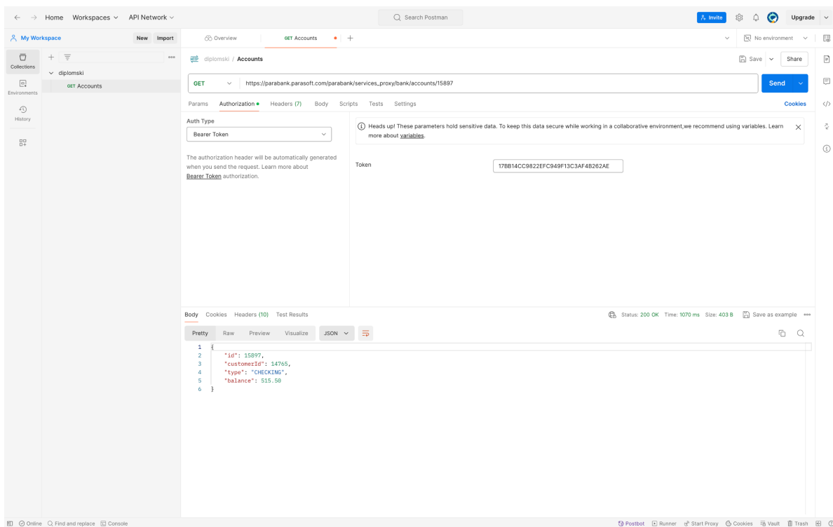
Slika 2.3. Sučelje Postman-a.
