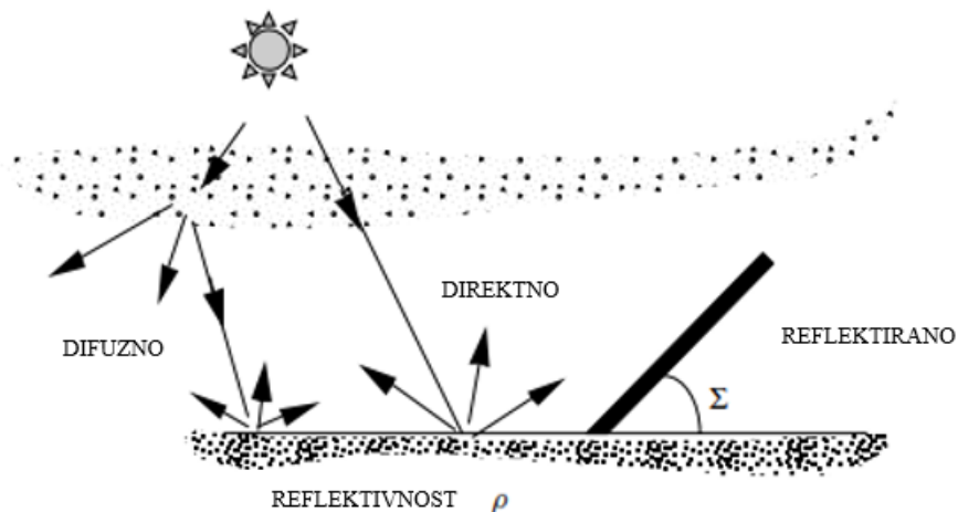
Slika 3.5. Tlo reflektira zračenje jednakim intenzitetom u svim smjerovima [12]
