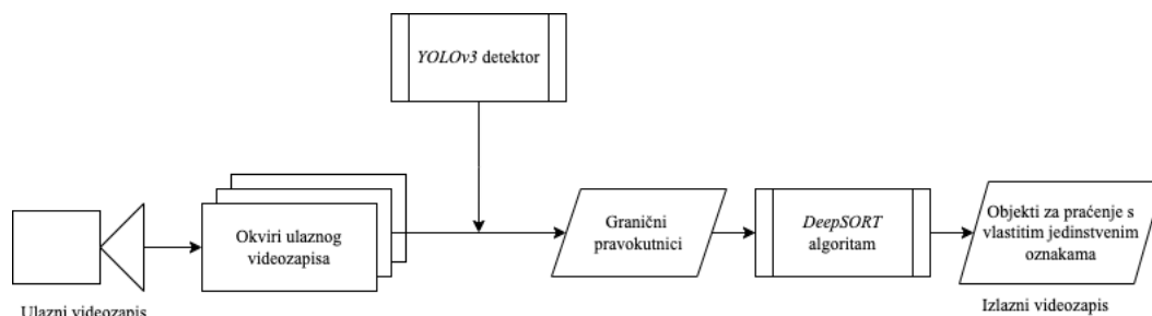
Sl. 2.7. Princip rada rješenja predstavljenog u radu [13]
