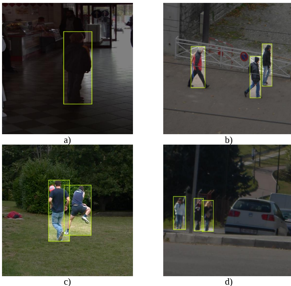
Sl. 3.3. Primjeri slika s označenim pješacima iz INRIA skupa podataka [19]
