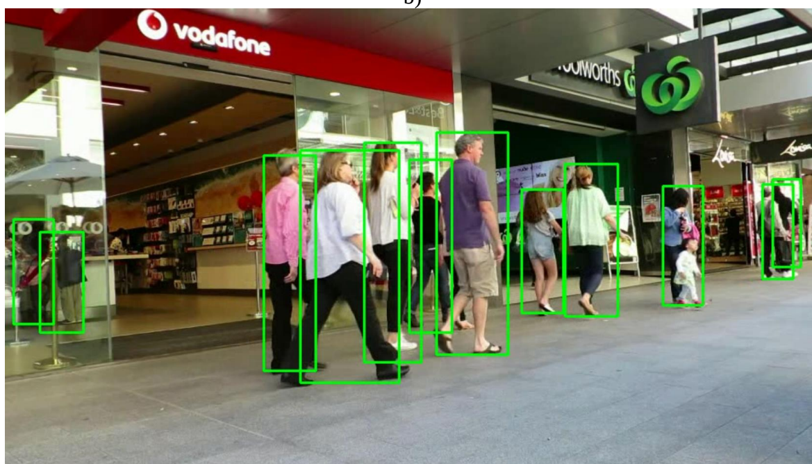
Sl. 3.16. Tri uzastopna okvira izlaznog videozapisa algoritma za detekciju i praćenje pješaka s SORT algoritmom
