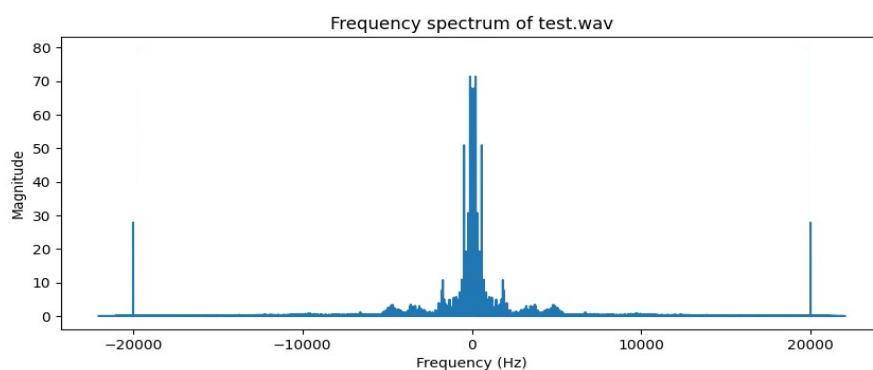
Slika 3.12. Prikaz frekvencijskog spektra signala nezadovoljavajuće magnitude
