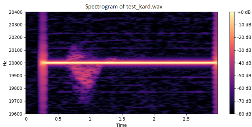
Slika 3.17. Spektrogram reflektiranog signala u kardioidnom načinu rada mikrofona
