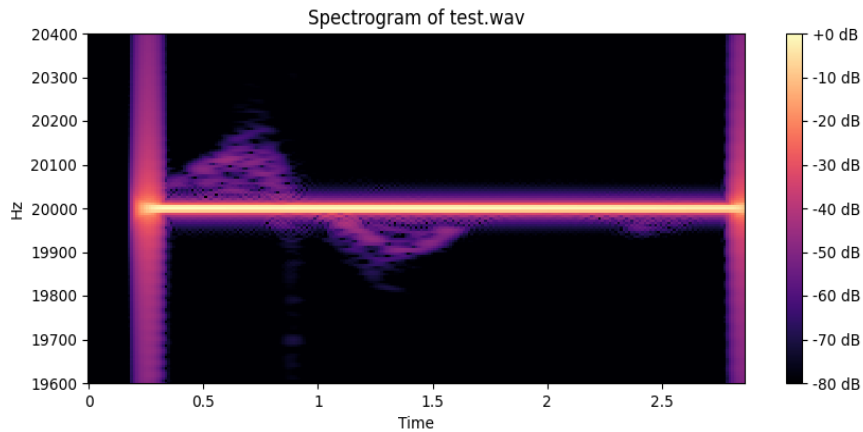
Slika 3.18. Spektrogram neželjenog reflektiranog signala
