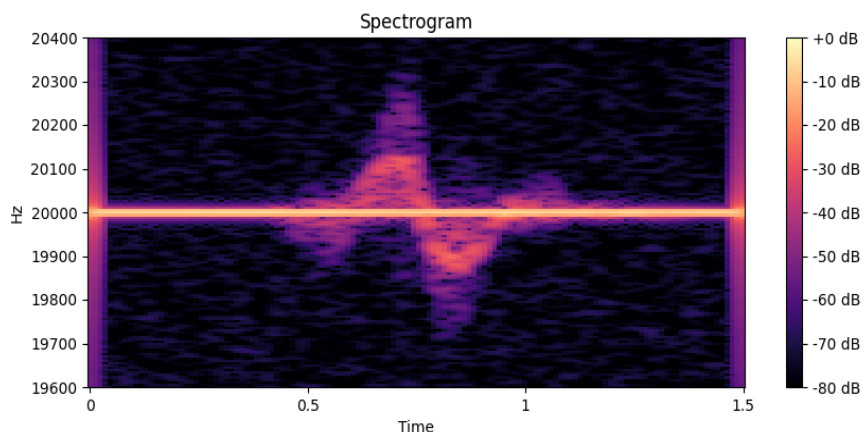
Slika 3.6. Spektrogram reflektiranog signala, vidljiv je Dopplerov pomak
