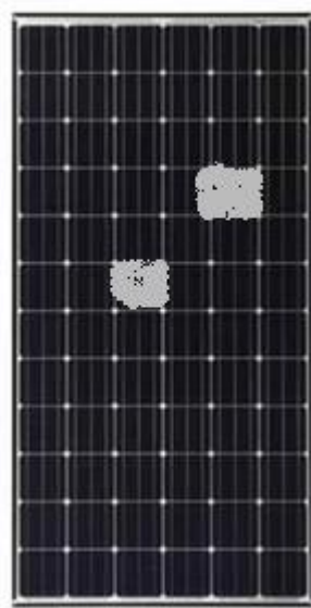
Slika 6.15. Zasjenjenje modula Panasonic VBHN240SE10 uzrokovano ptičjim izmetom
