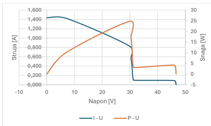
Slika 6.14. I-U i P-U karakteristike modula Panasonic VBHN240SE10 pri zasjenjenju desnog stupca modula.
