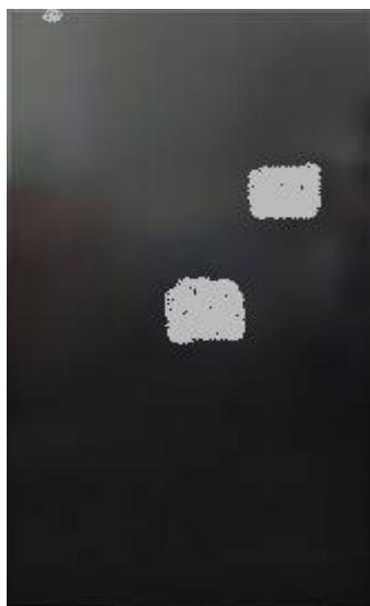
Slika 6.26. Zasjenjenje modula Solar Frontier SF-150 uzrokovano ptičjim izmetom.
