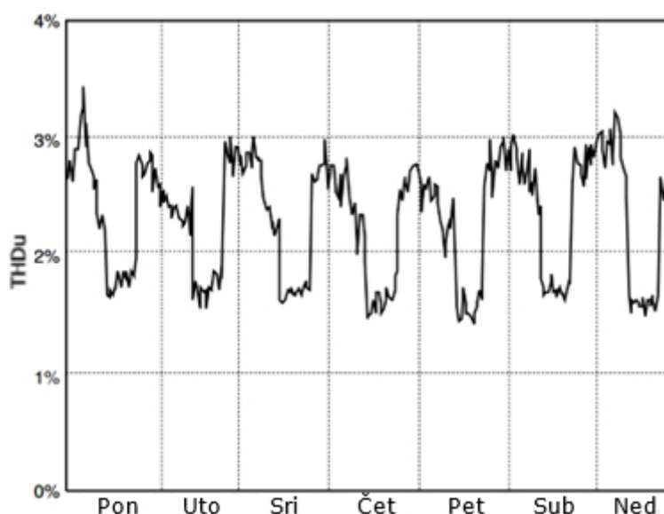
Slika 4.4. Promjena THD-a tijekom tjedna [1]
