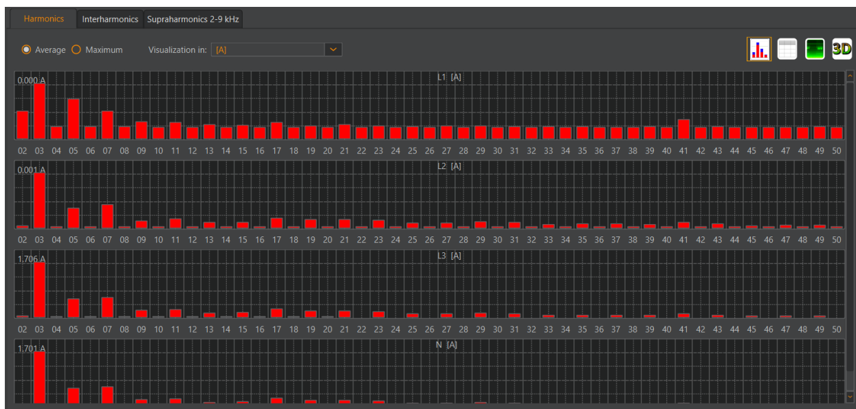
Slika 5.9. Dijagram strujnih harmonika pri jednofaznom punjenju
