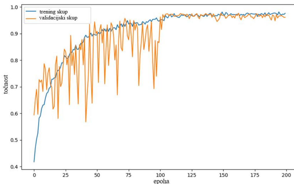
Slika 3.4. Krivulja točnosti na trening i validacijskom skupu kroz epohe tro-klasnog modela
