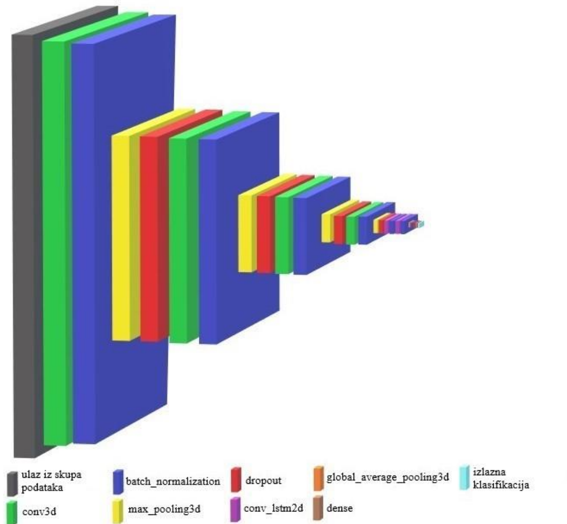
Slika 3.2. Vizualizirani prikaz korištene arhitekture LRCN mreže
