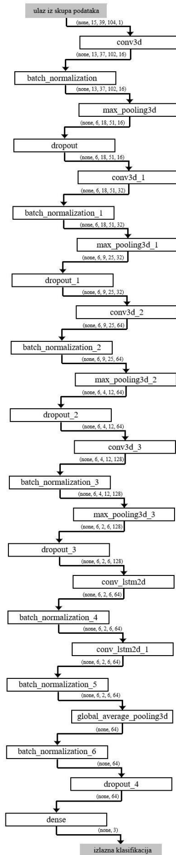
Slika 3.1. Prikaz arhitekture LRCN mreže korištene u ovome radu
