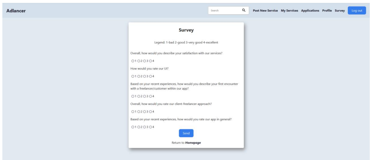
Slika 4.23. Prikaz upitnika
