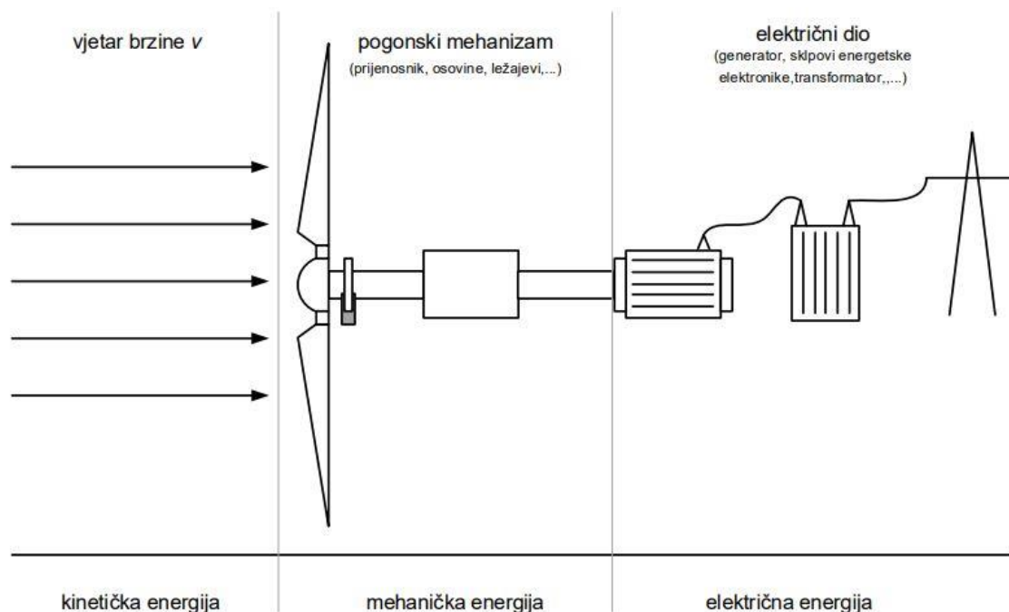
Slika 2.1 Lanac pretvorbi energije kod vjetroeletkrana [2]
