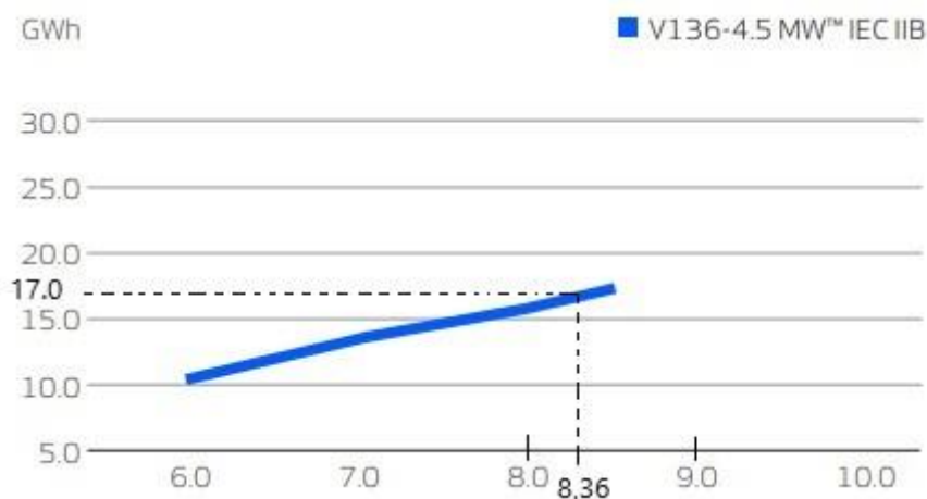
Slika 4.6 Godišnji prihodi električne energije u ovisnosti o brzini vjetra za navedeni proizvod [15]
