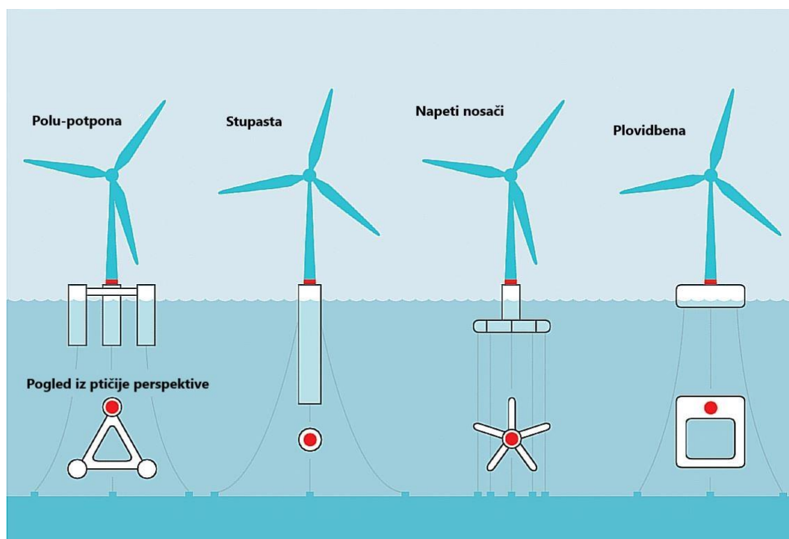
Slika 2.3 Vrste plutajućih vjetroturbina [4]
