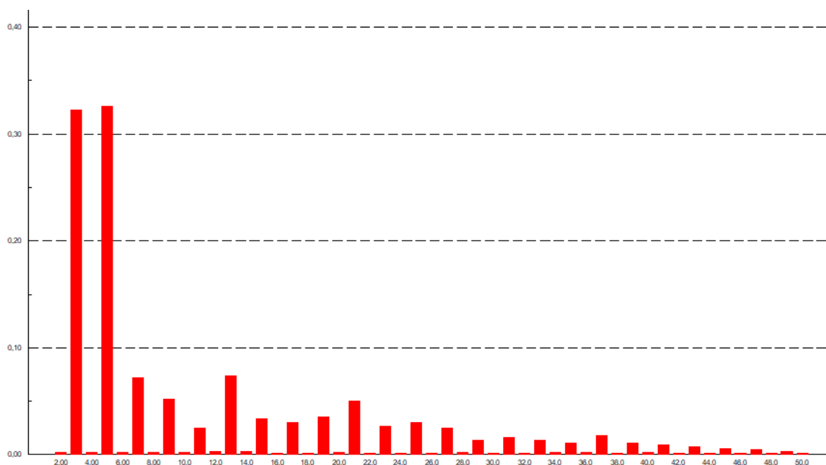
Slika 7.2. Harmonijski spektar struje za Slučaj 1
