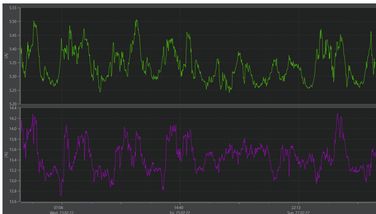
Slika 6.15. Dijagram efektivne struje (zeleno) i TDD (ljubičasto)
