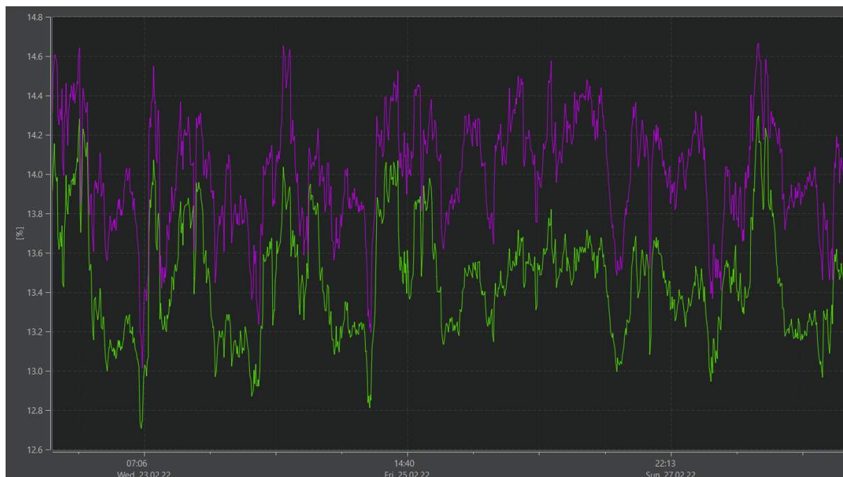
Slika 6.14. Dijagram THD-a struje (ljubičasto) i TDD (zeleno) u postotcima
