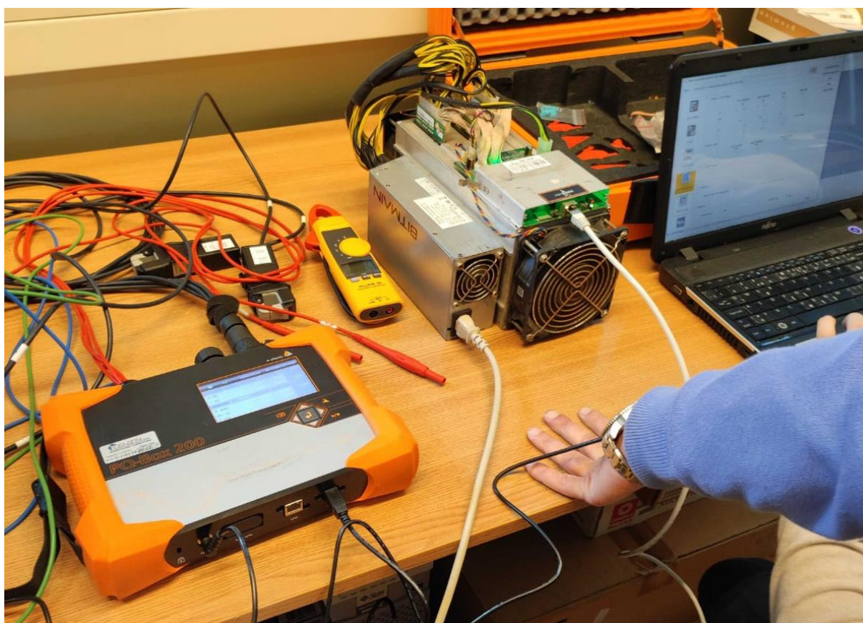
Slika 6.1. Mjerenje utjecaja ASIC sklopovlja na kvalitetu električne energije u zgradi FERIT- a
