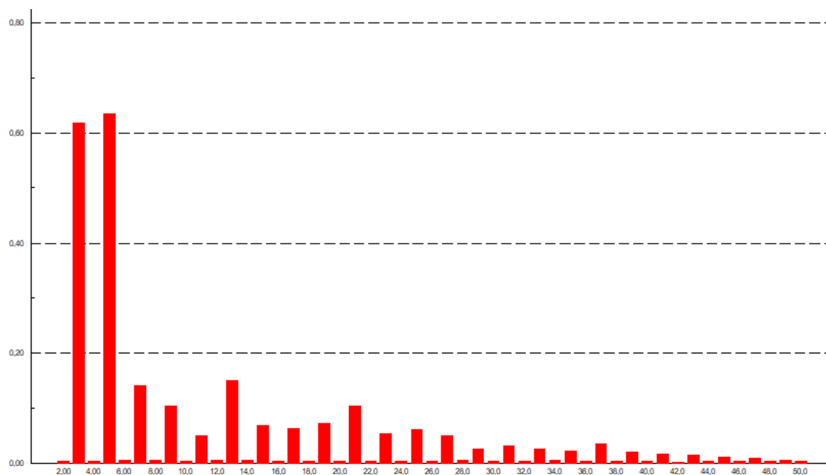
Slika 7.8. Harmonijski spektar struje za Slučaj 3
