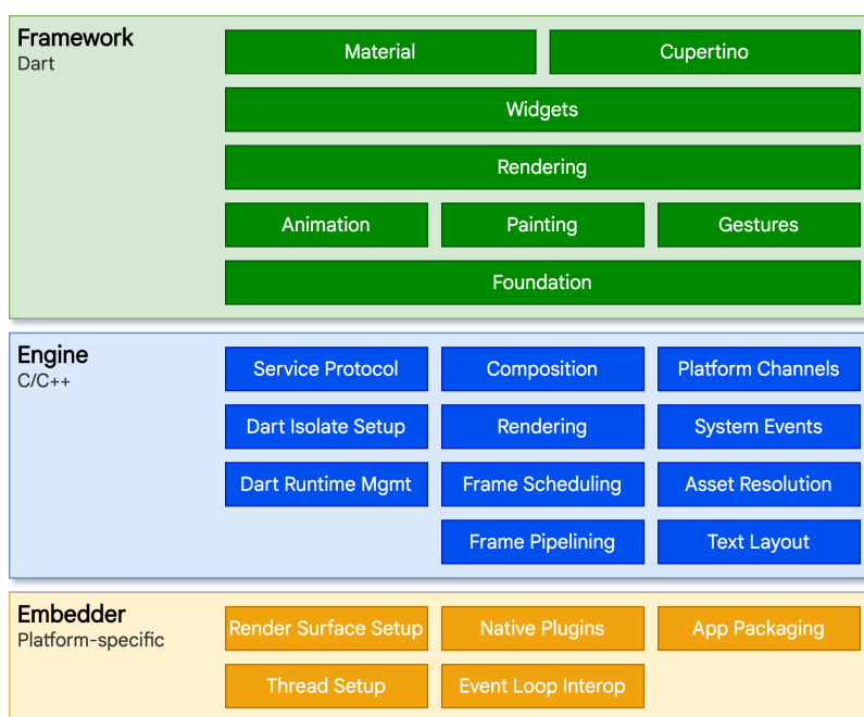
Slika 2.3: Flutter arhitektura [10]
