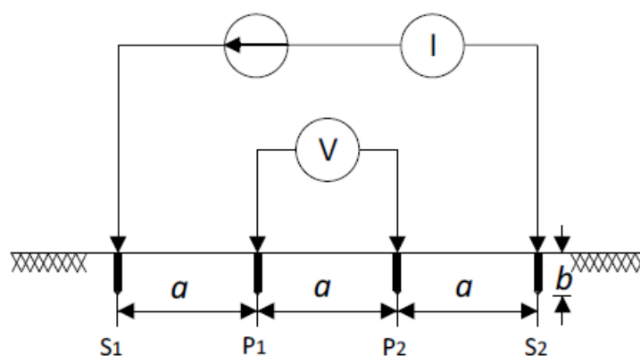
Slika 2.3. Wennerova metoda [2]
