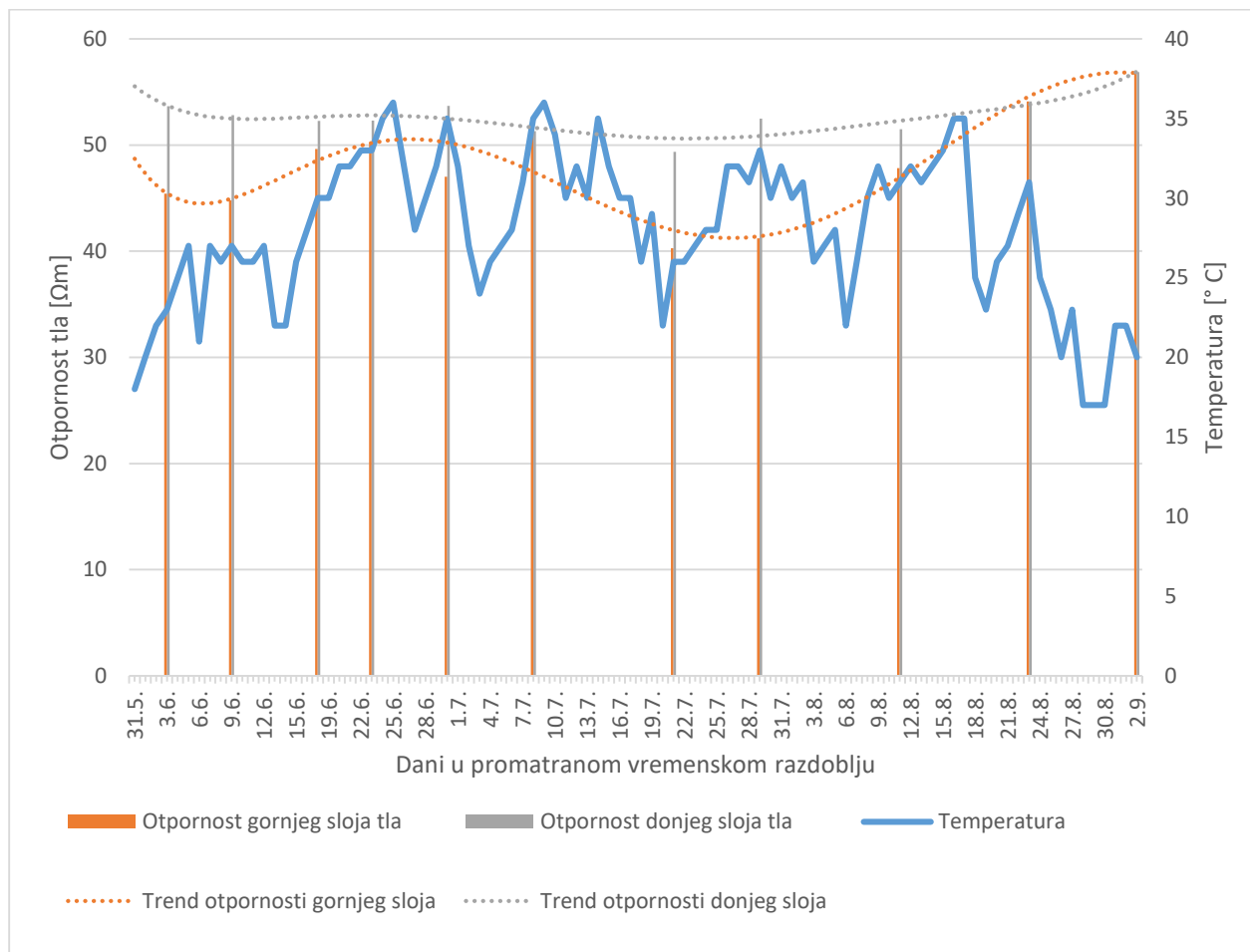
Slika 4.18. Odnos temperature i otpornosti tla u promatranom vremenskom razdoblju
