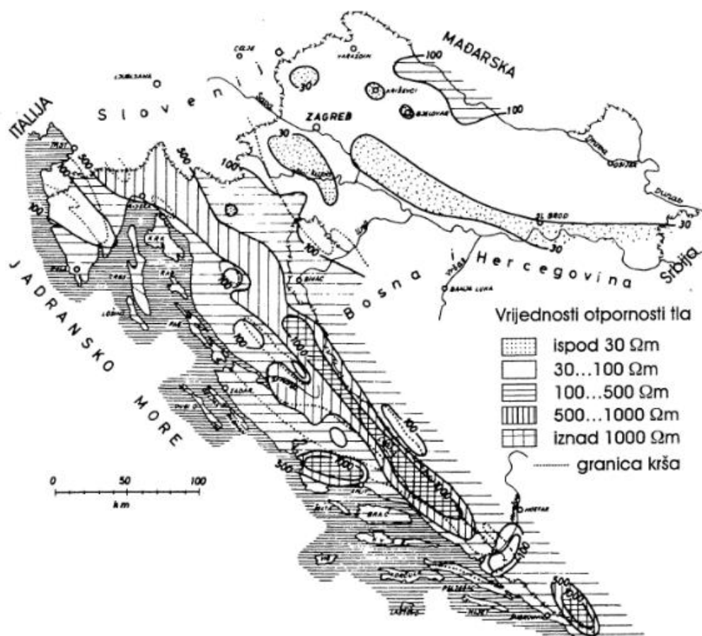
Slika 2.1. Vrednovanje električne otpornosti tla na području Hrvatske [1]
