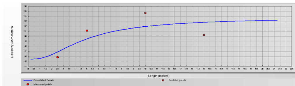
Slika 4.5. Grafička analiza: Dvoslojno tlo (prvo mjerenje)
