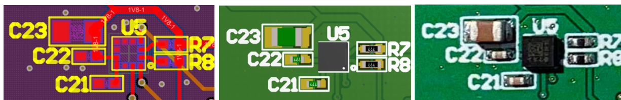
Slika 3.16. Prikaz sheme, 3D modela te stvarne pločice sustava za detekciju pokreta.
