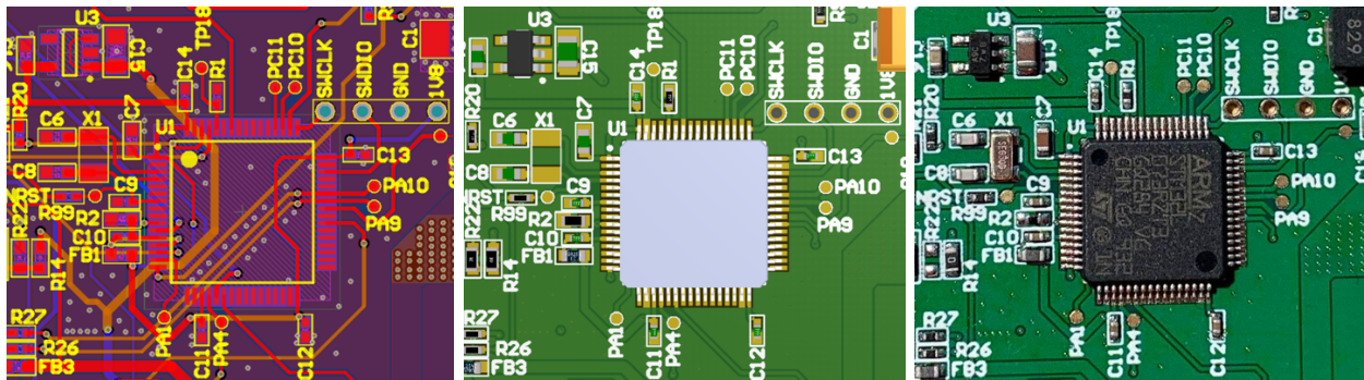
Slika 3.21. Prikaz sheme, 3D modela te stvarne pločice mikroupravljača.
