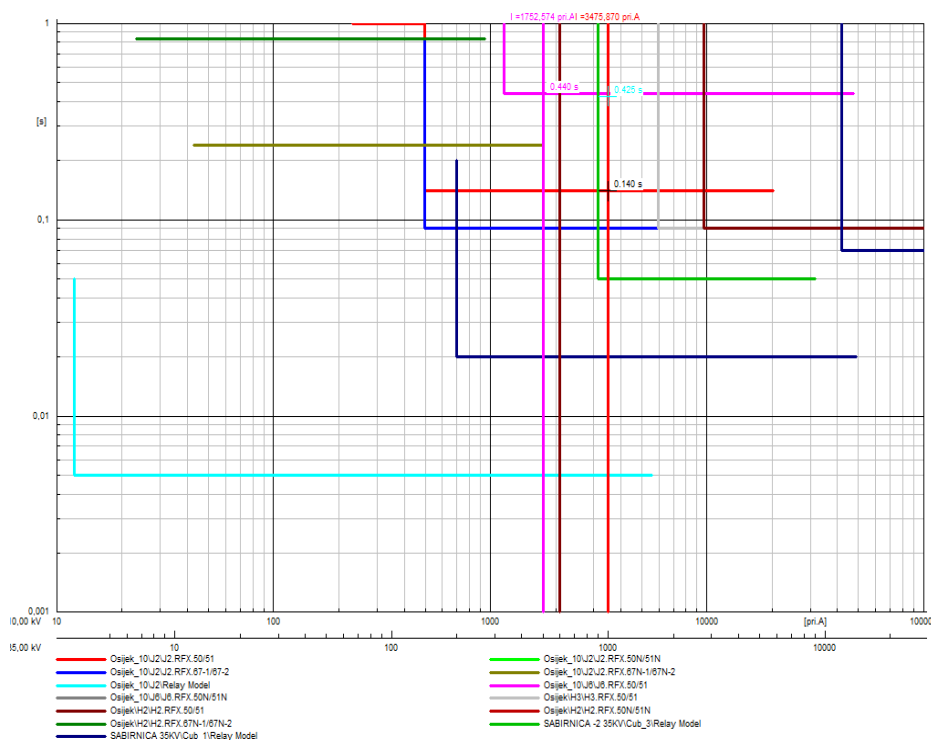
Slika 6.22. Koordinacija mreže za troljni kratki spoj
